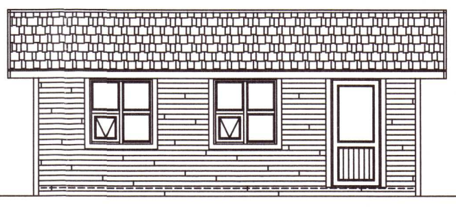
ÚTLIT SUÐUR
