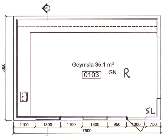
GRUNNMYND
