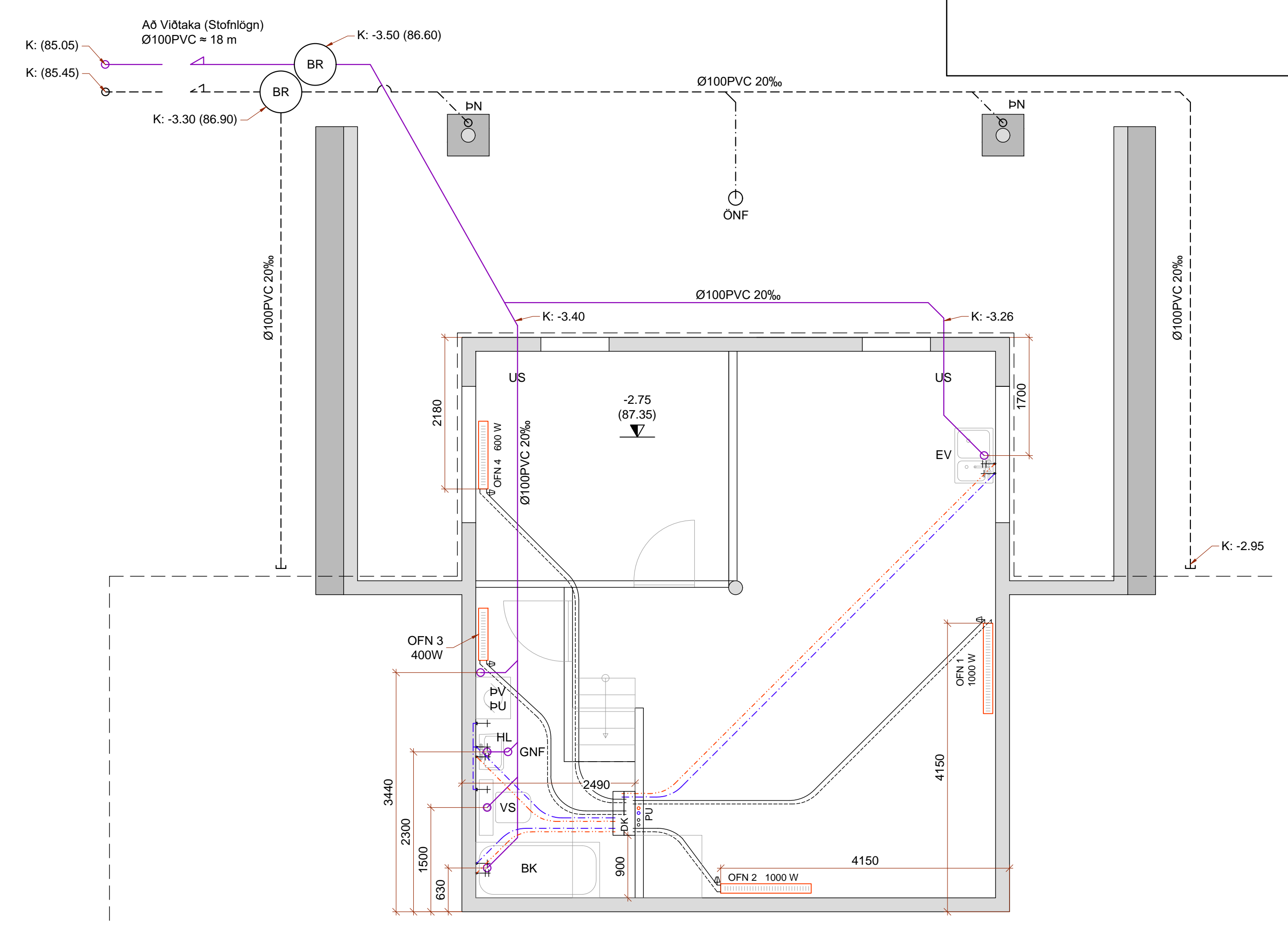
GRUNNMYND - KJALLARI Mkv. 1:50
