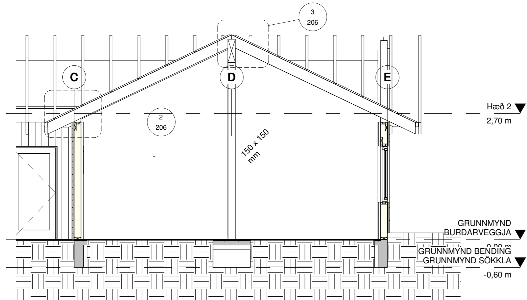
1 PVERSKURÐUR Í MIÐJU HÚSS 1 : 50
