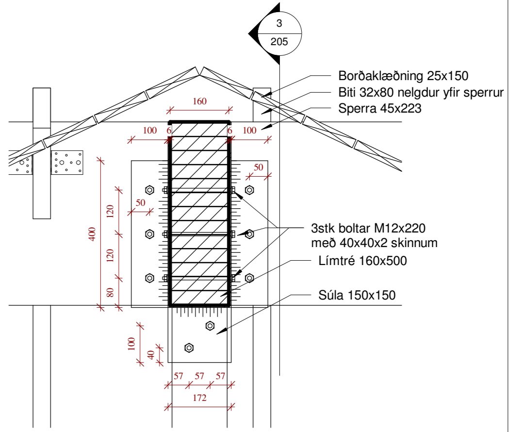
2 SKURÐUR Í ÞVERBITA Í MÆNI 1 : 10
