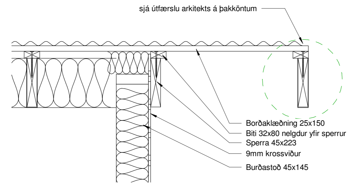
4 SKURÐUR Í ÞAKGAFL 1 : 10
