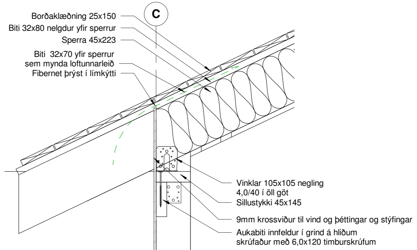
2 DEILI Í ÞAKKANTA 1 : 10
