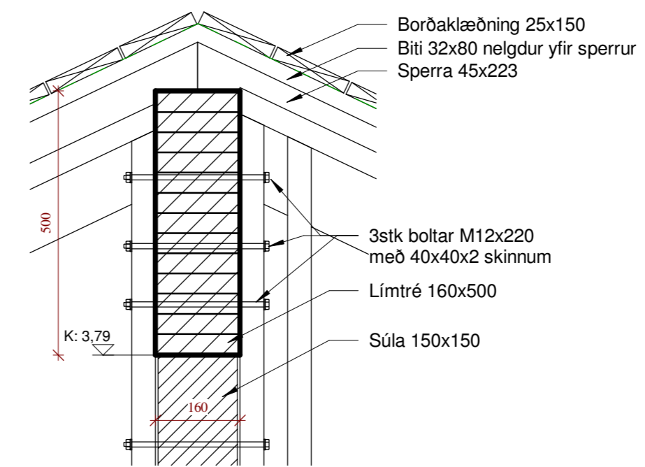
5 FESTING BITA Í MÆNI 1 : 10
