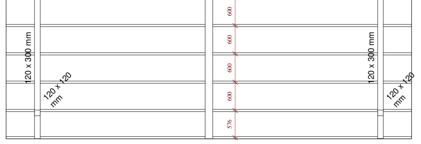
1 GRUNNMYND BURÐARVEGGJA 1 : 50
