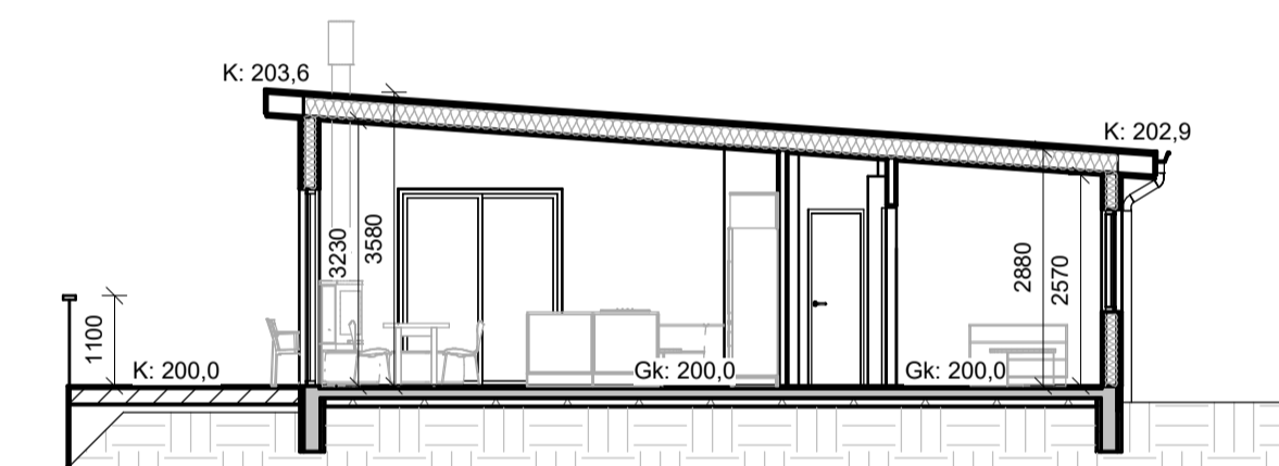
02 SNID A101 1 : 100
