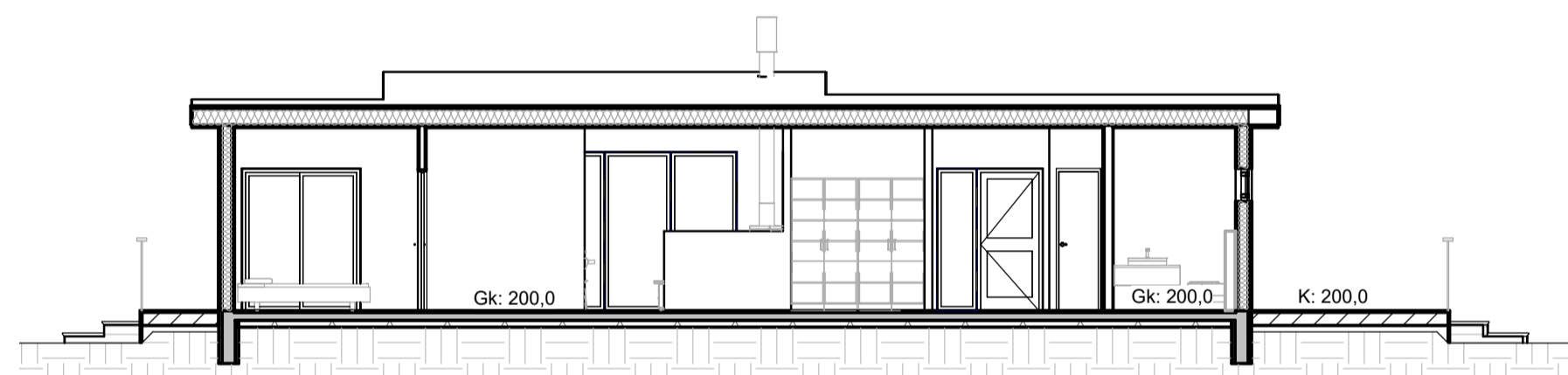
01 SNID A101 1 : 100
