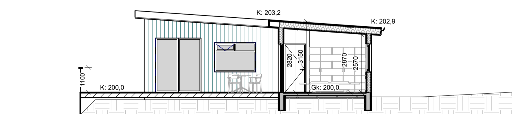
03 SNID A101 1 : 100
