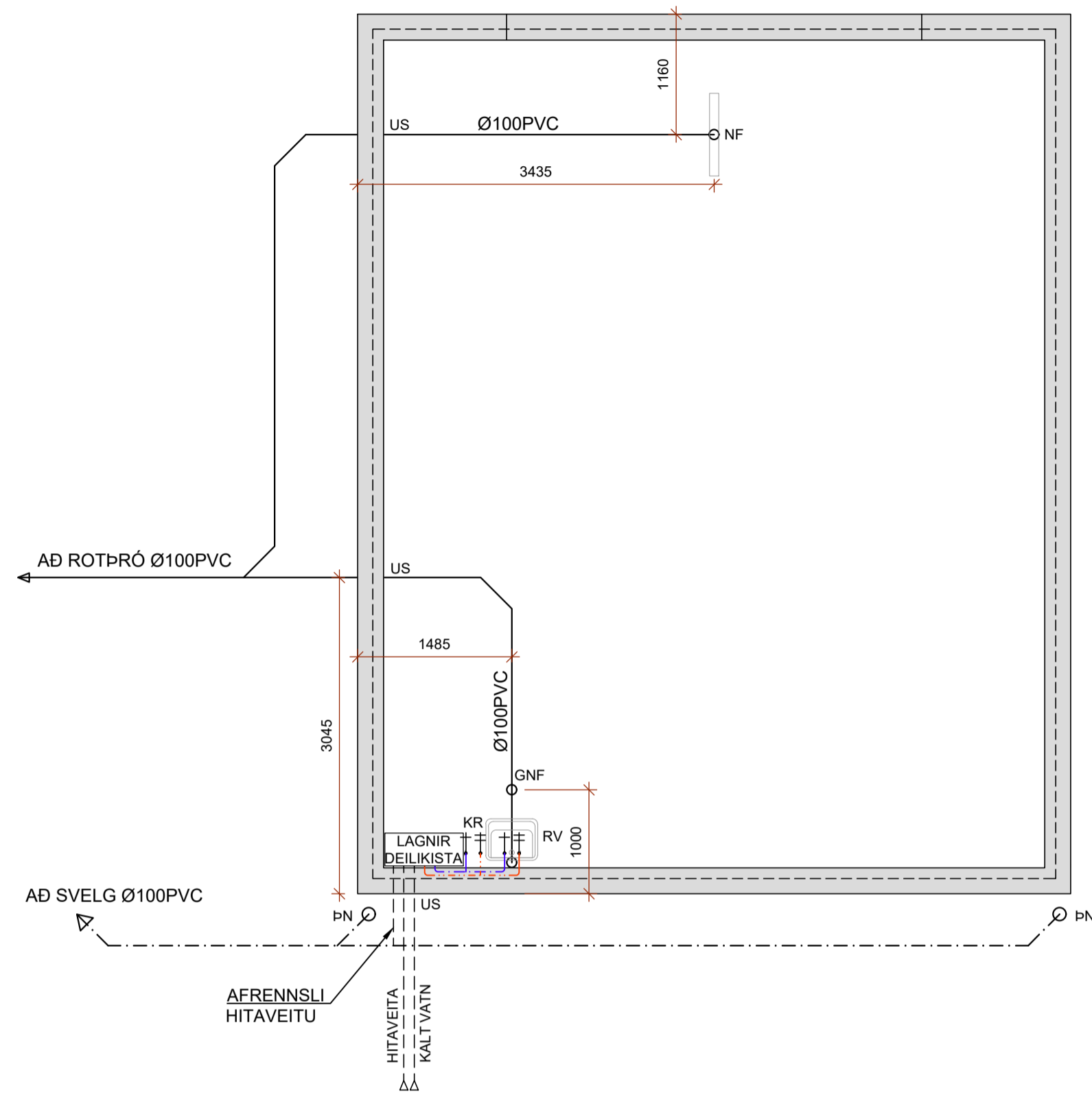
GRUNNMYND - FRÁRENNSLI OG NEYSLUVATN Mkv. 1:50
