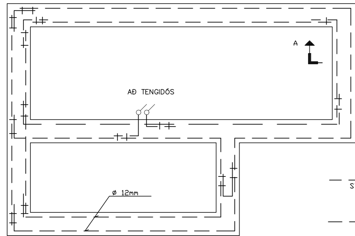
GRUNNMYND SÖKKULVEGGJA
