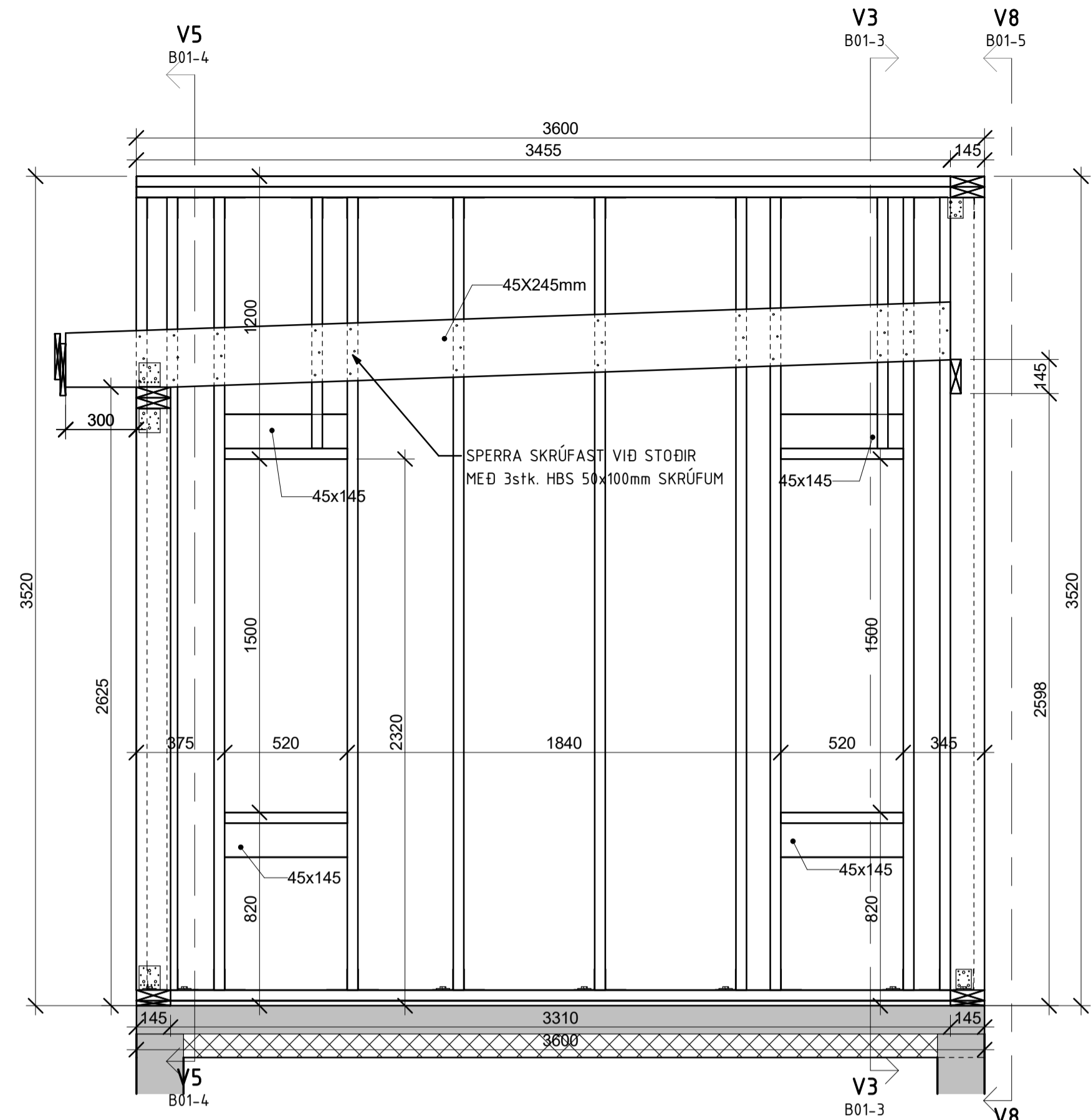
VEGGUR V4 1 : 20
