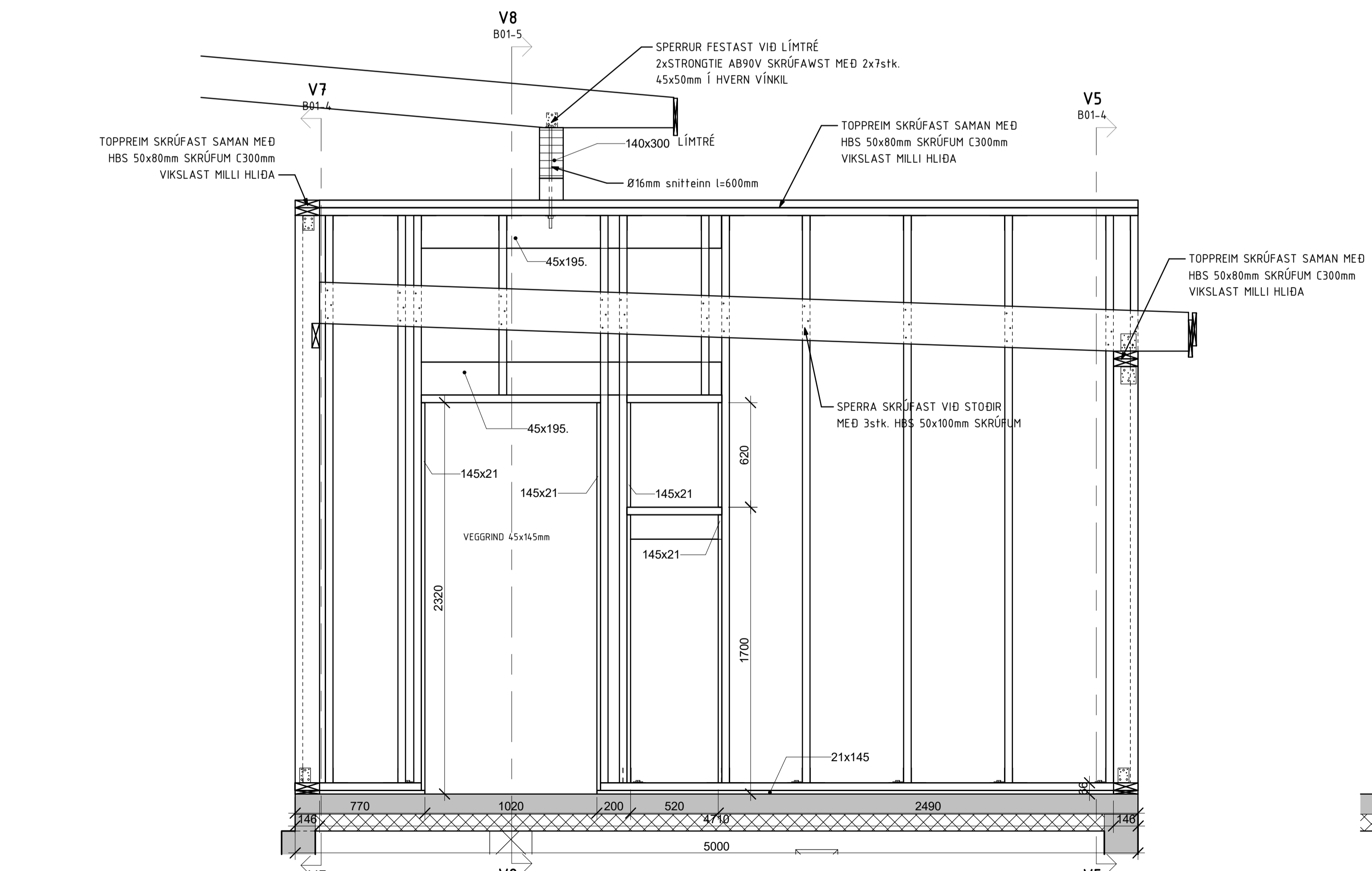
VEGGUR V6 1 : 20
