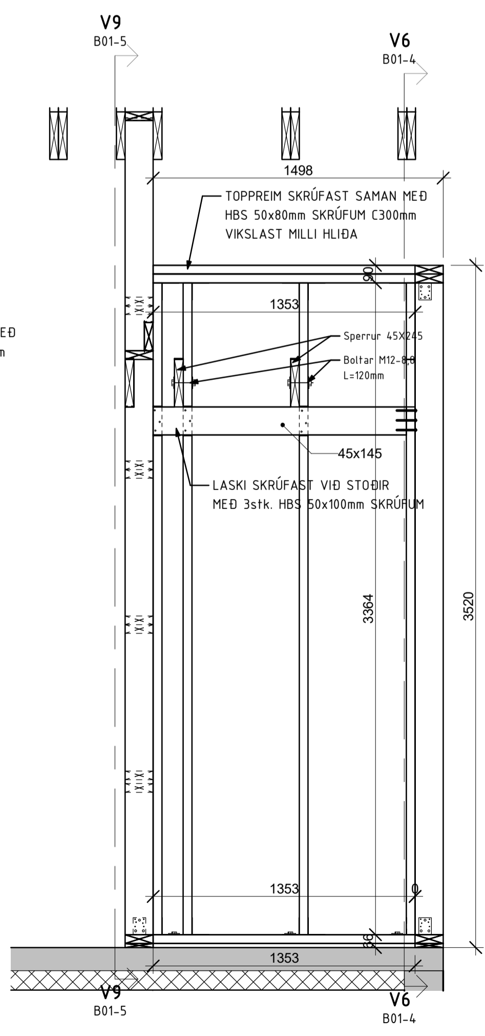
VEGGUR V7 1 : 20
