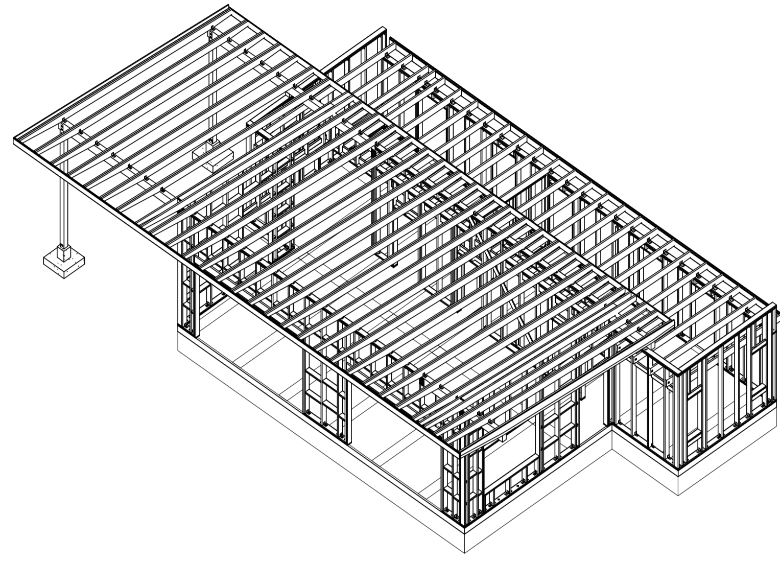
ÞRÍVÍDD 1
