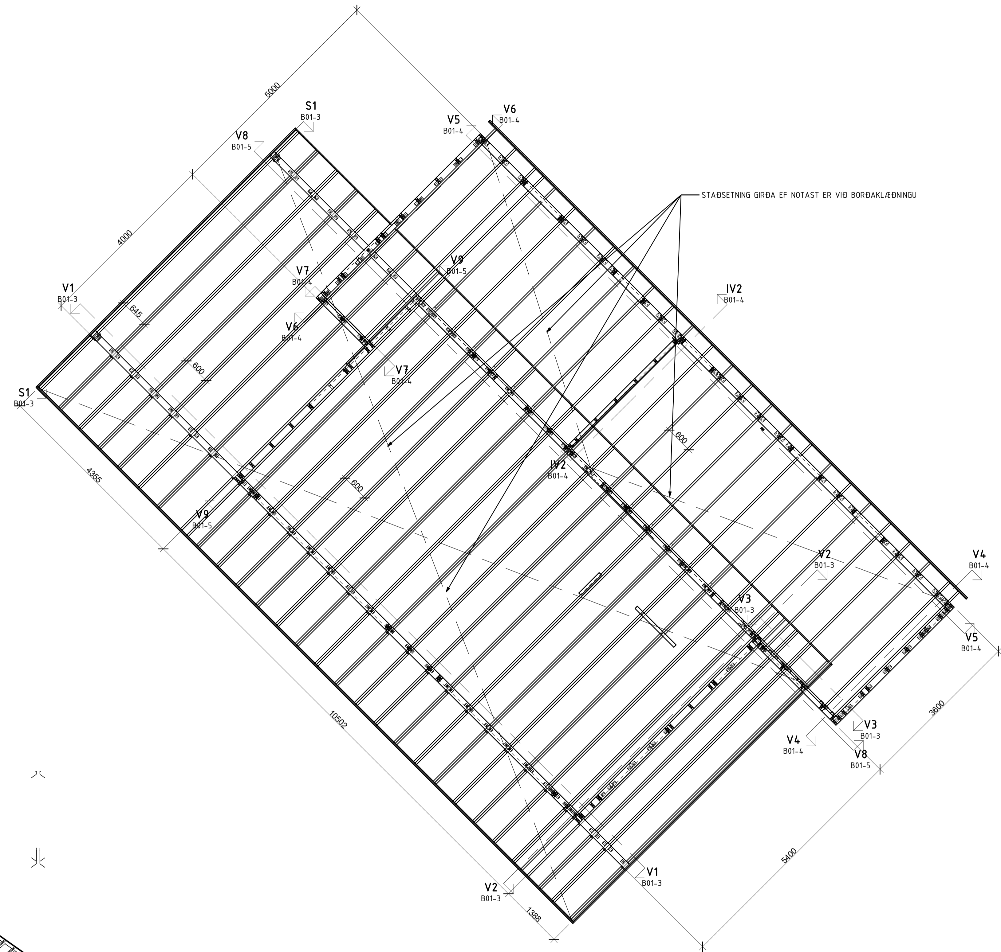
GRUNNMYND HÆÐAR 1 : 50
