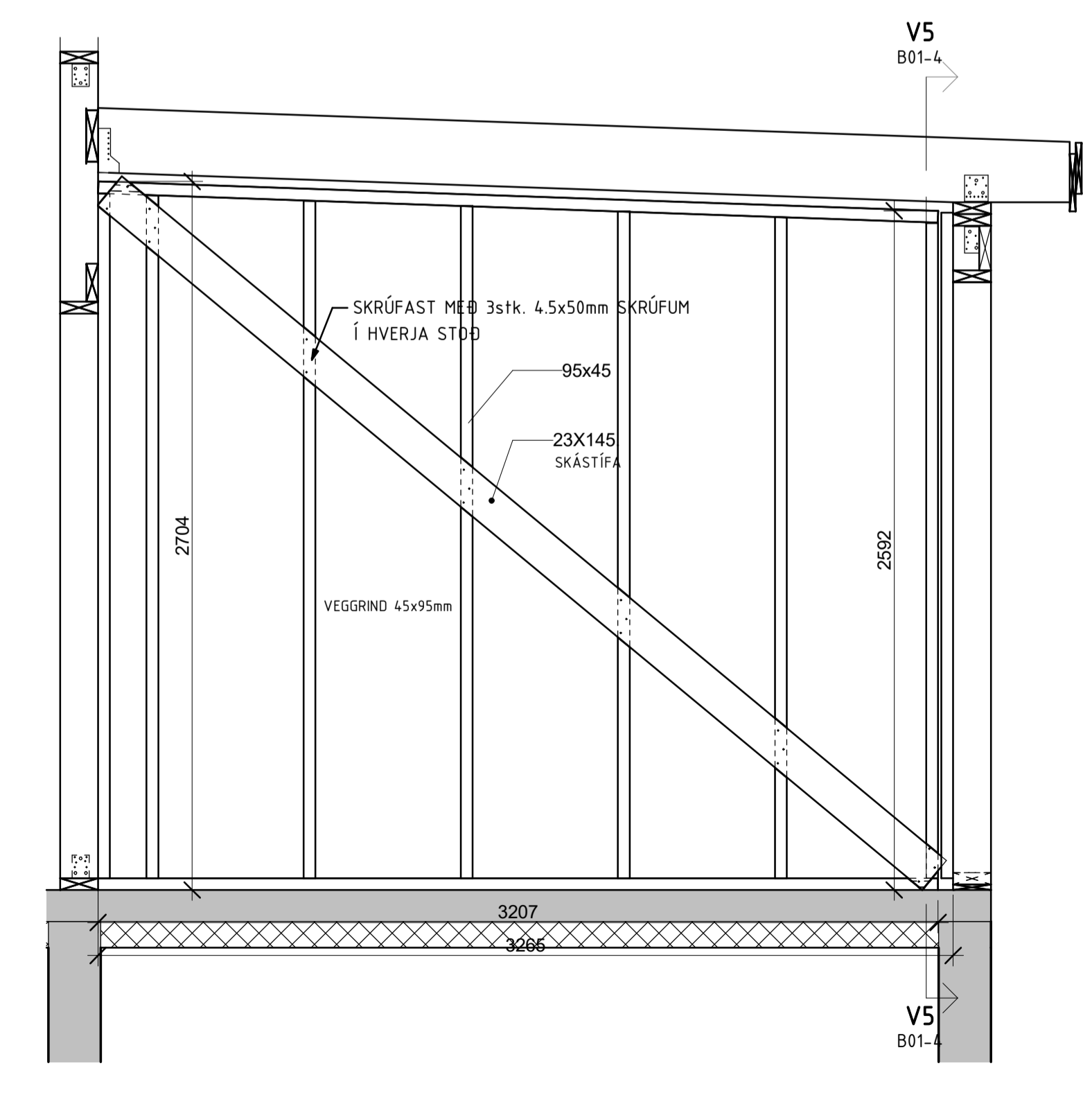
VEGGUR IV2 1 : 20
