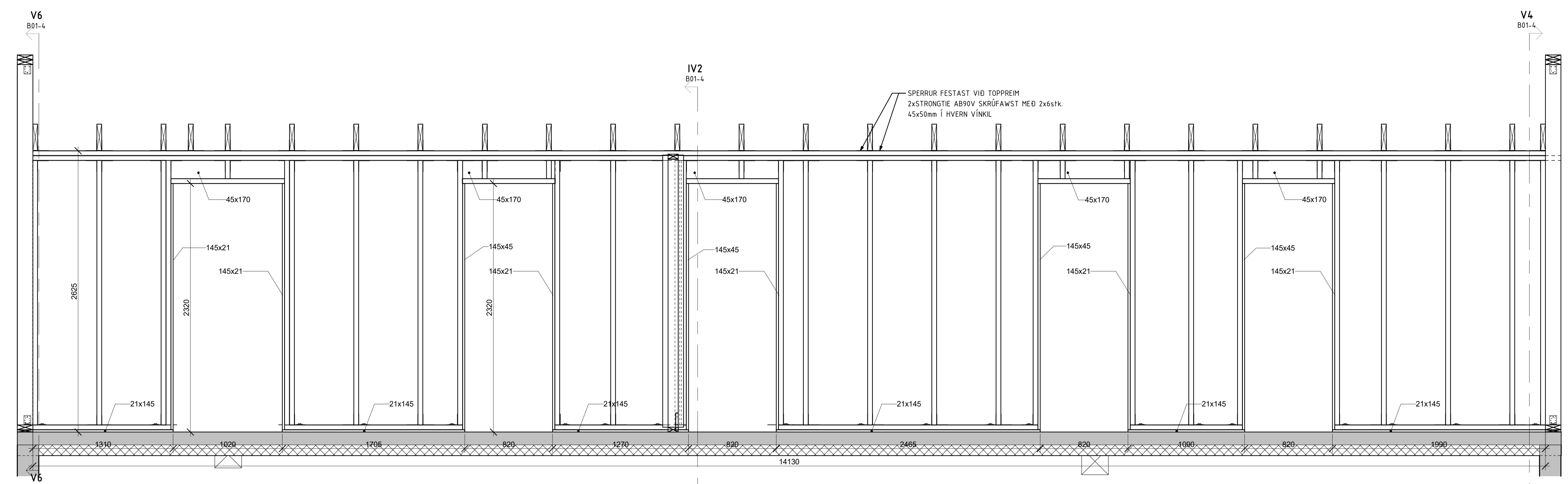
VEGGUR V5 1 : 20
