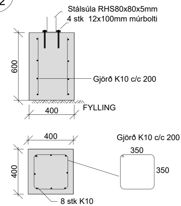
C SNIÐ C-C 1:20
