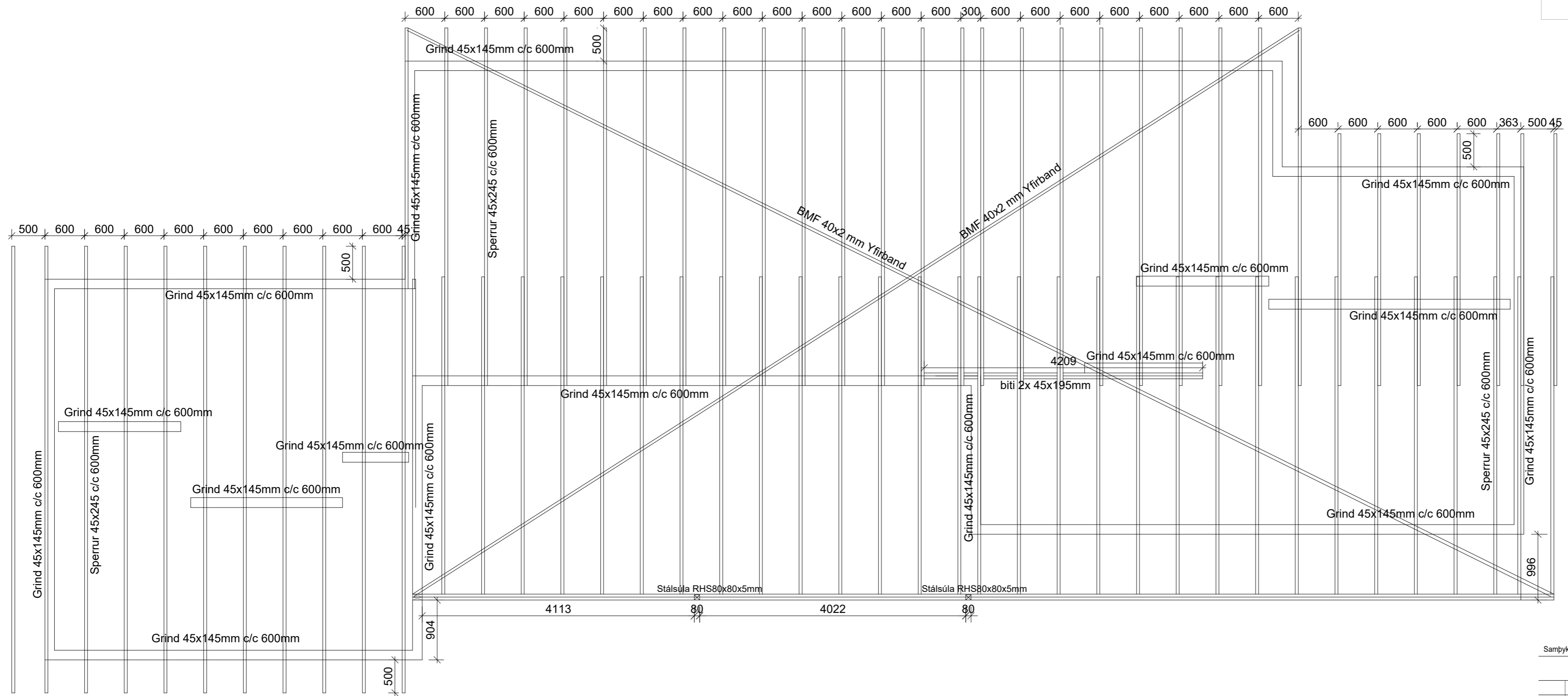
Sperrur og bitar þak 1:50
