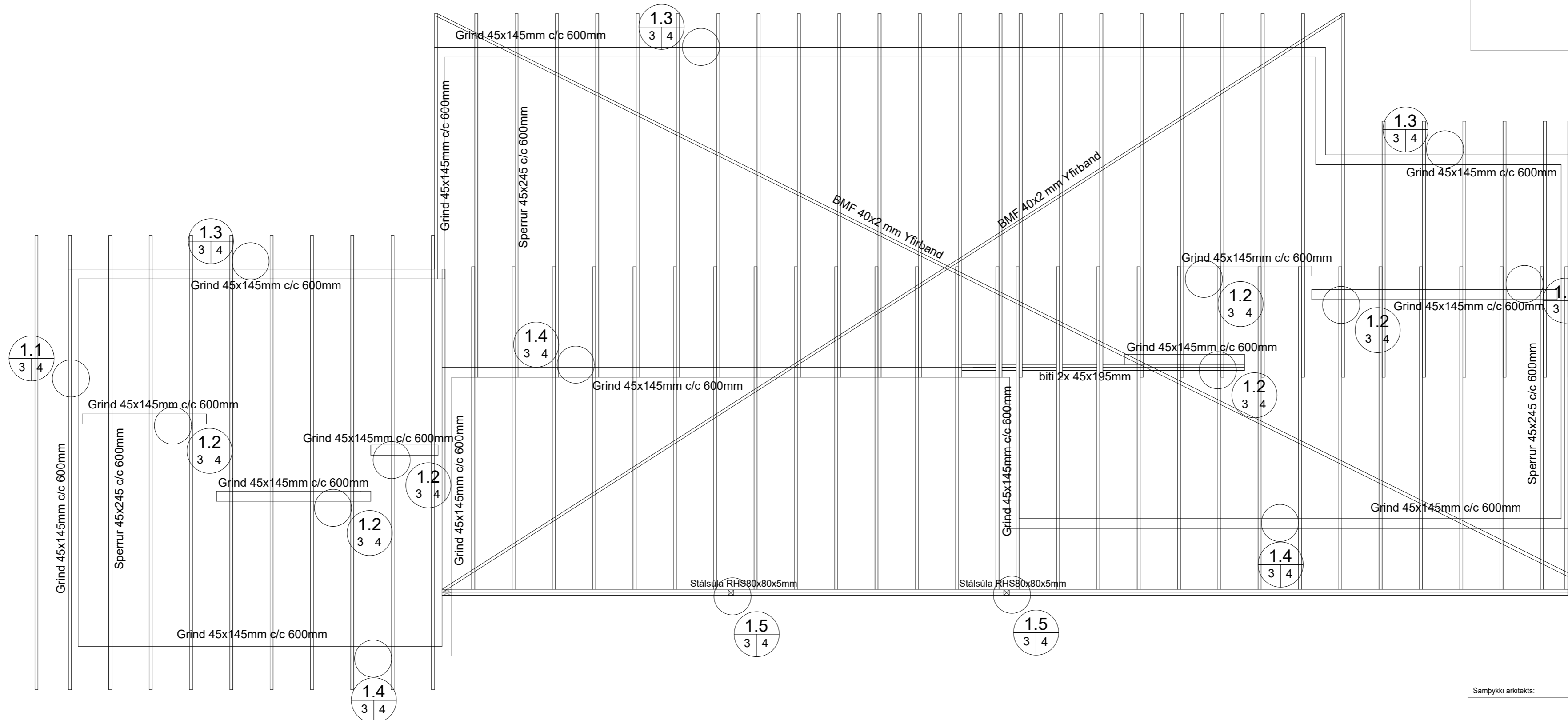
Grunnmynd og sperruplan 1:50
