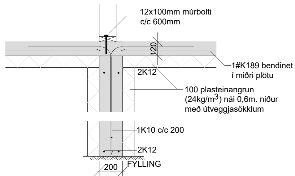
B SNIÐ B-B 1:20
