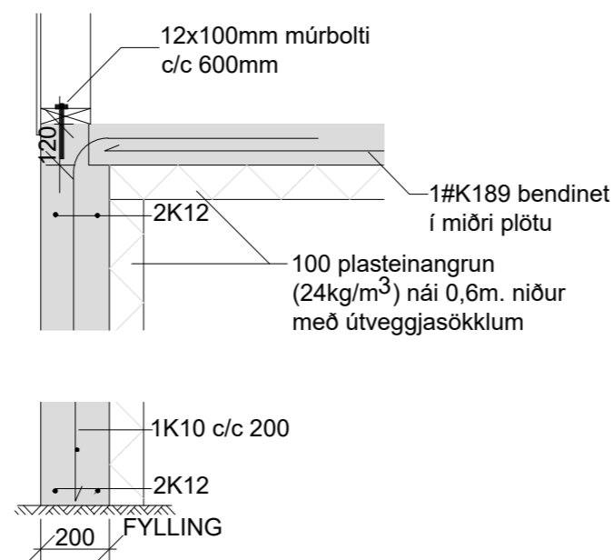
A SNIÐ A-A 1:20
