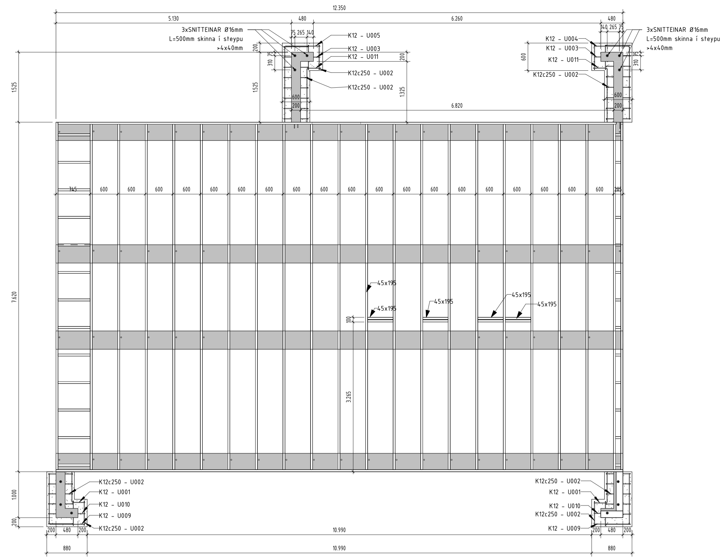
GRUNNMYND, SÖKKLAR 1 : 50
