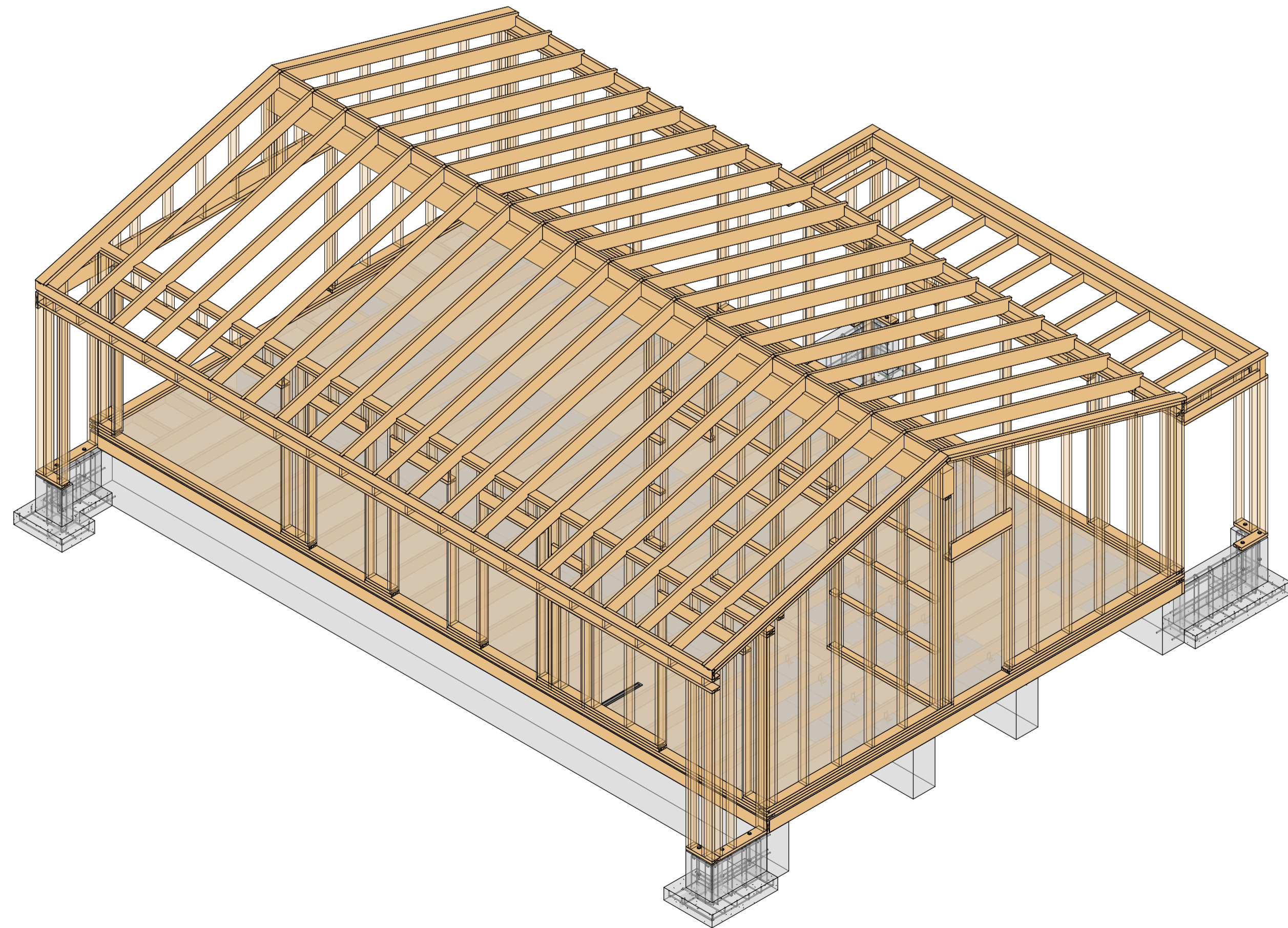
RÚMMYND - BURÐARVIRKI 2.
