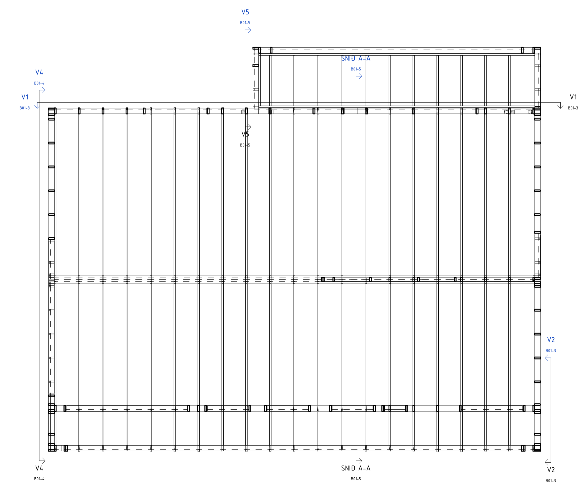
GRUNNMYND ÞAK 1 : 50
