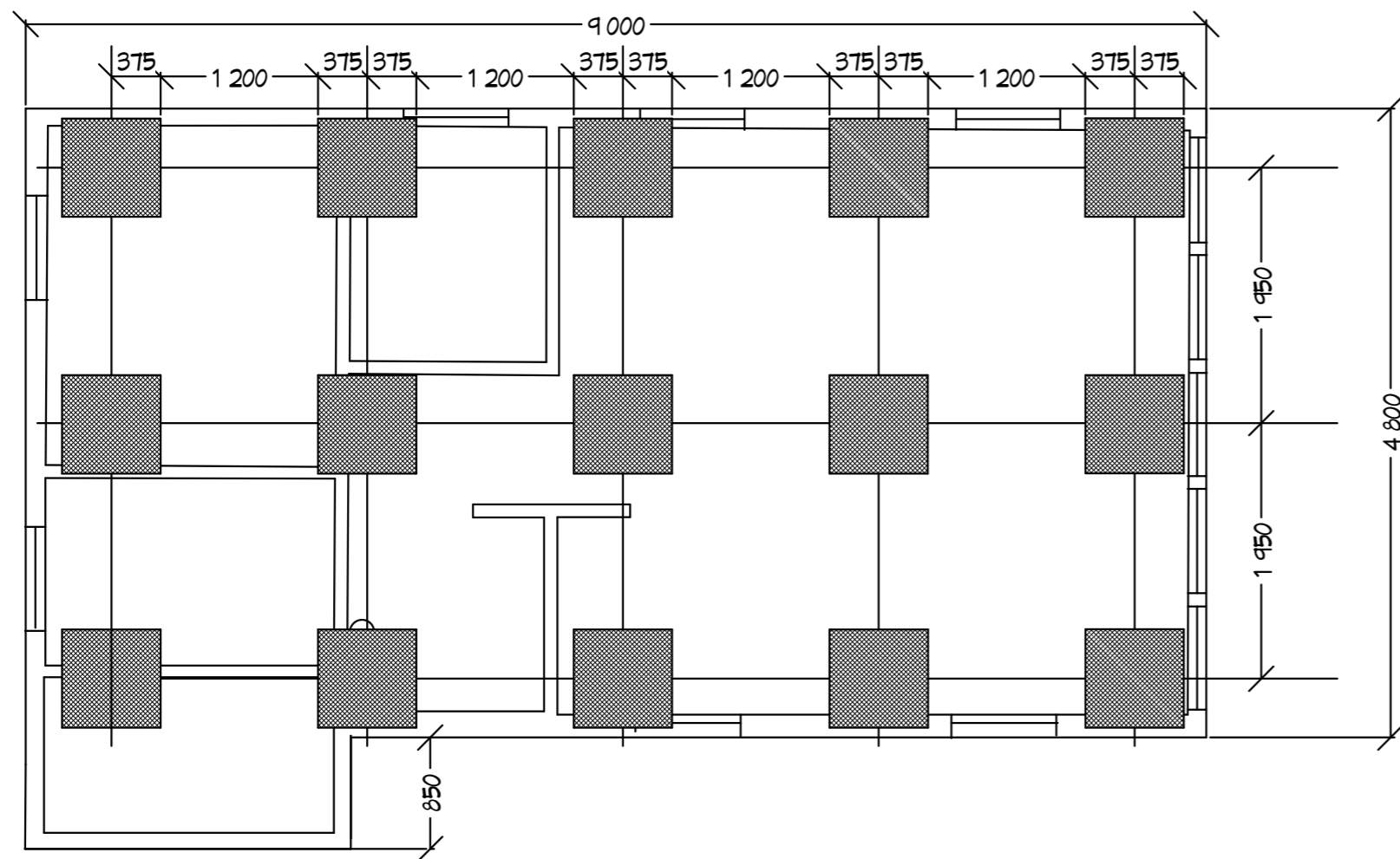
Steyptar undirstöður 750 x 750 x 300 , hvíla á þjappaðri fyllingu. Hæð kubbanna er 300 mm, bil á milli er 1200 mm
