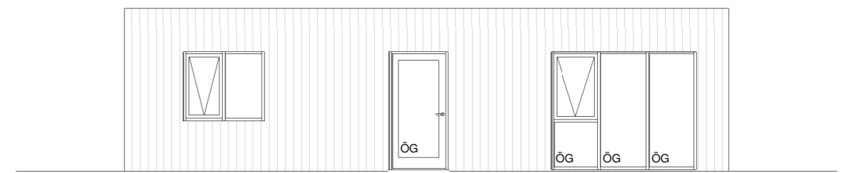
Norður 1 : 100
