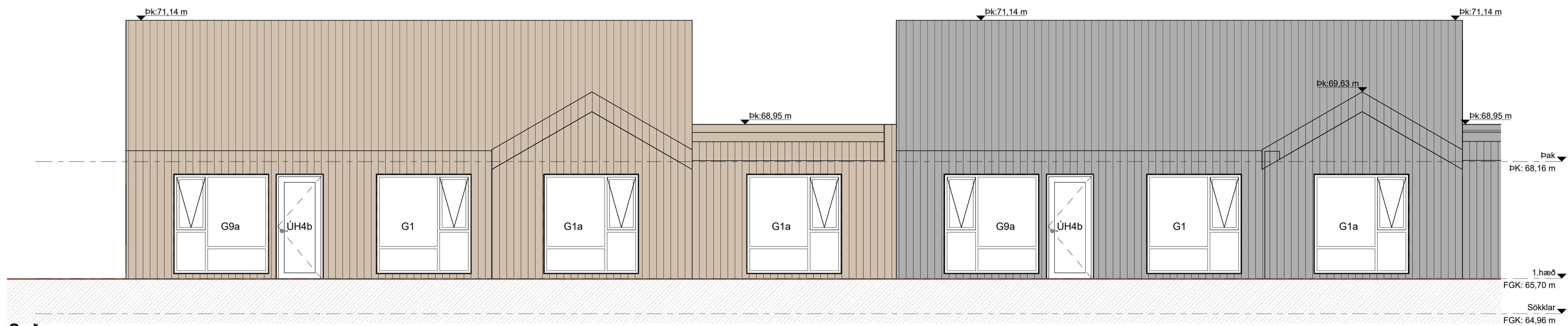
Suður mkv: 1 : 50
