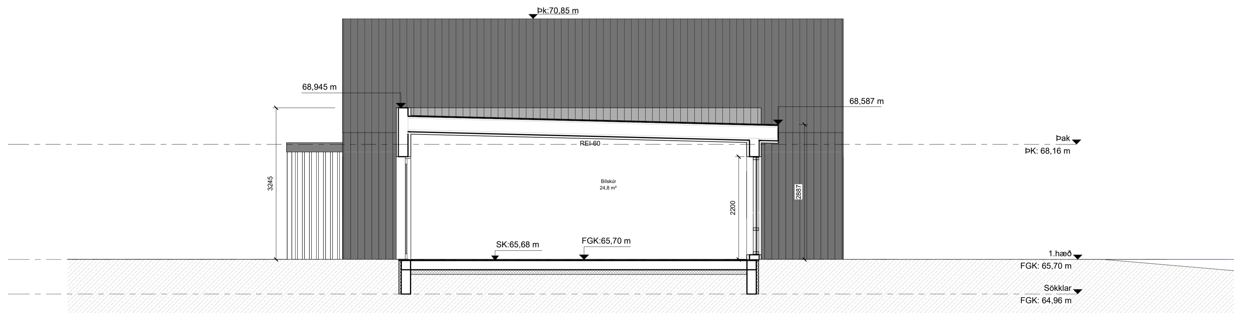
snið D-D Verkt. mkv: 1 : 50
