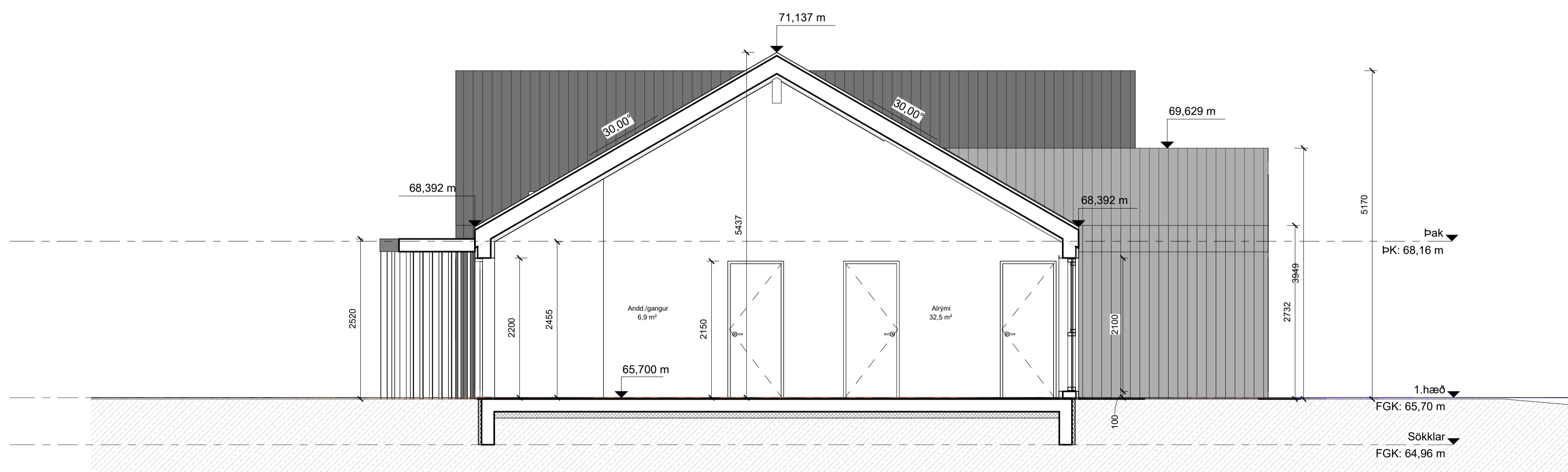
snið C-C Verkt. mkv: 1 : 50
