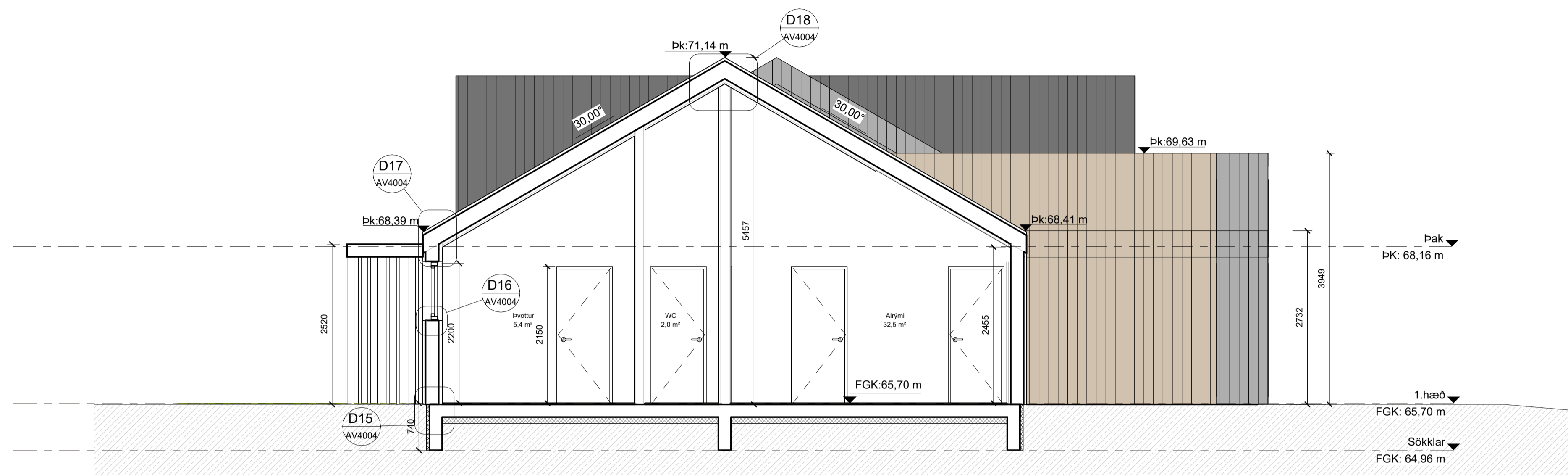
snið B-B Verkt. mkv: 1 : 50
