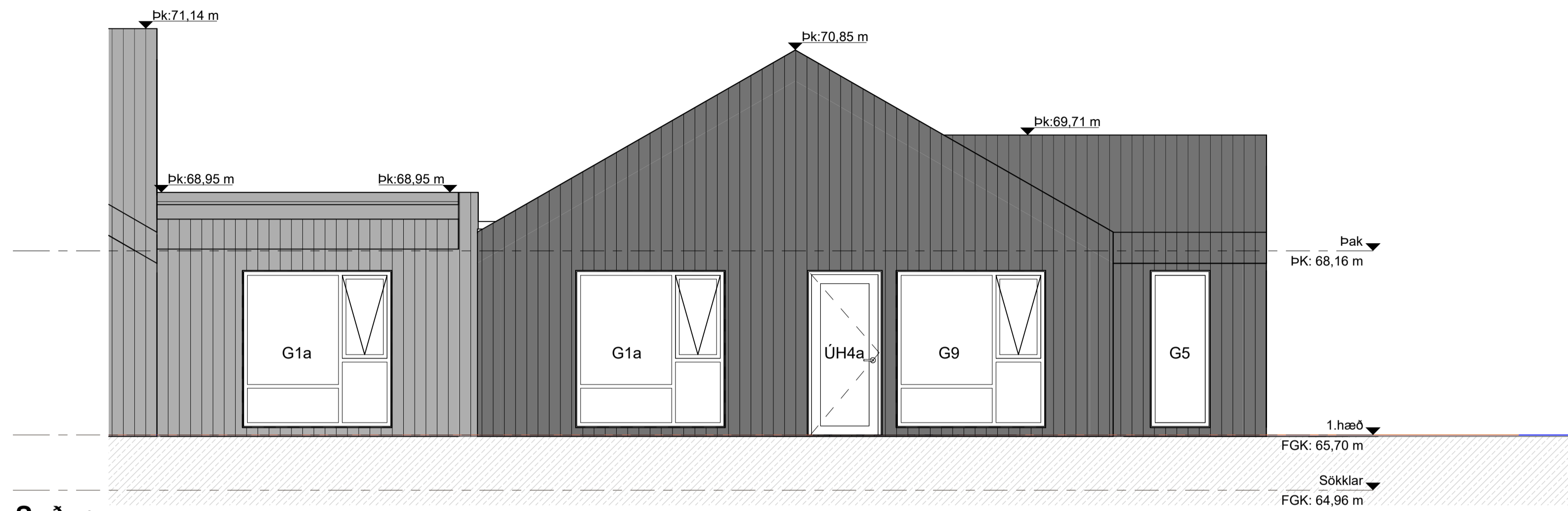
Suður mkv: 1 : 50
