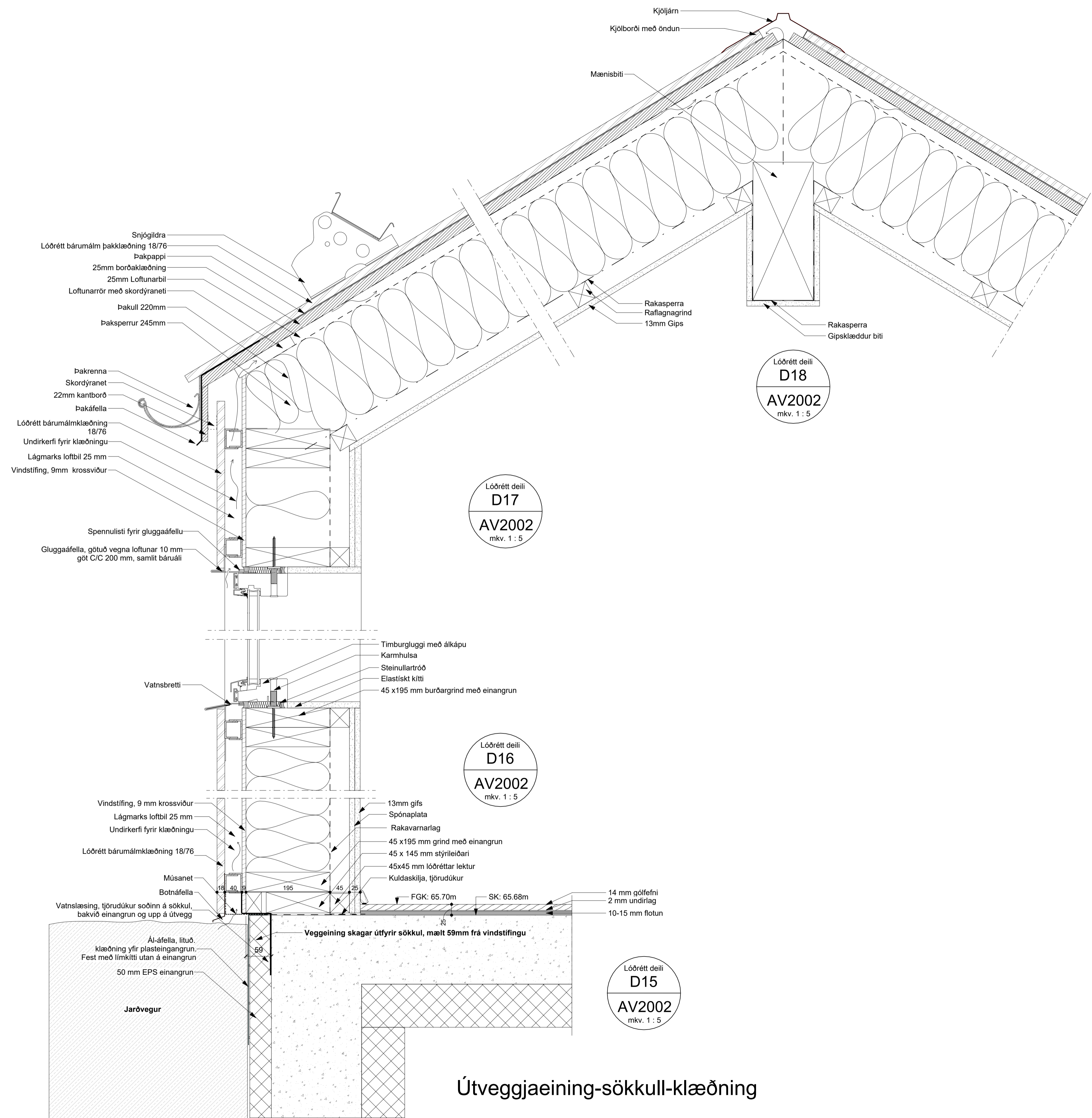
Deili lóðrétt - veggur - þak mkv: 1 : 5
