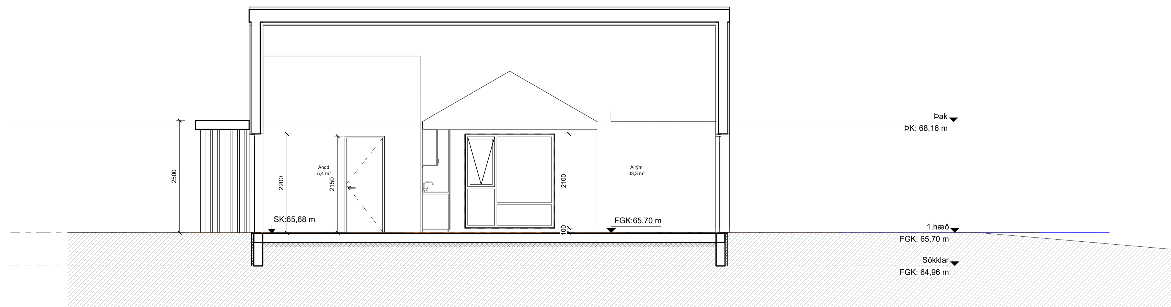
snið E-E Verkt. mkv: 1 : 50
