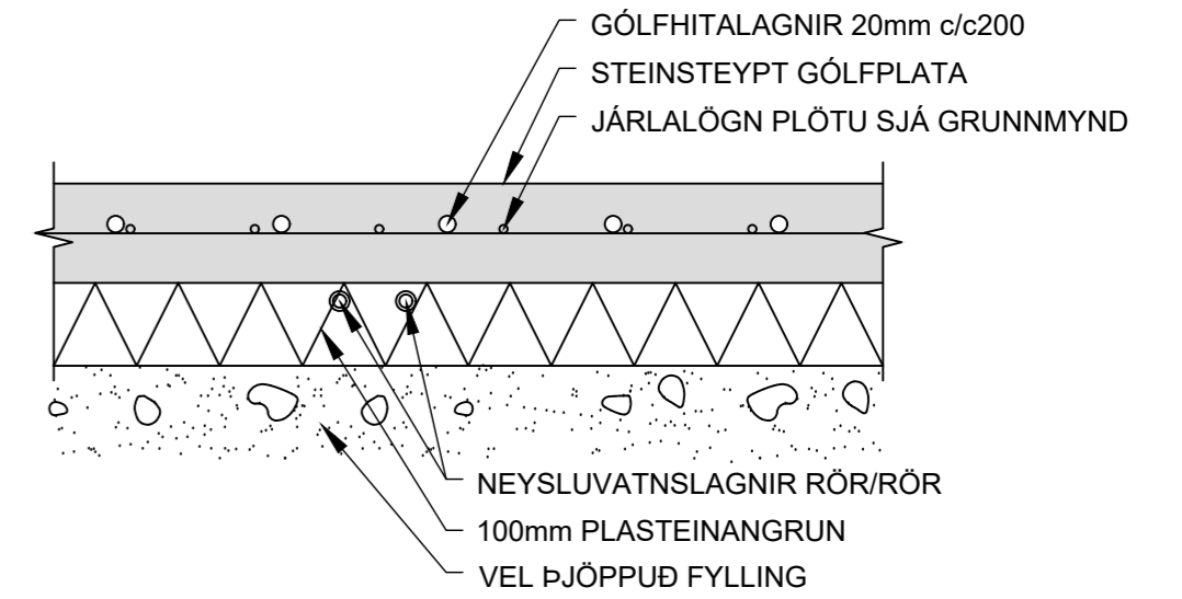
ALMENNT SNID Í GÓLFPLÖTU Á FYLLINGU NEYSLUVATNS OG GÓLFHITALAGNIR 1:10
