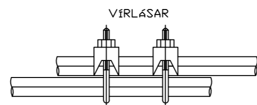
SAMTENGING STEYPUVEINA SETJA SKAL TVO VÍRLÁSA Á HVER SAMSKEYTI
