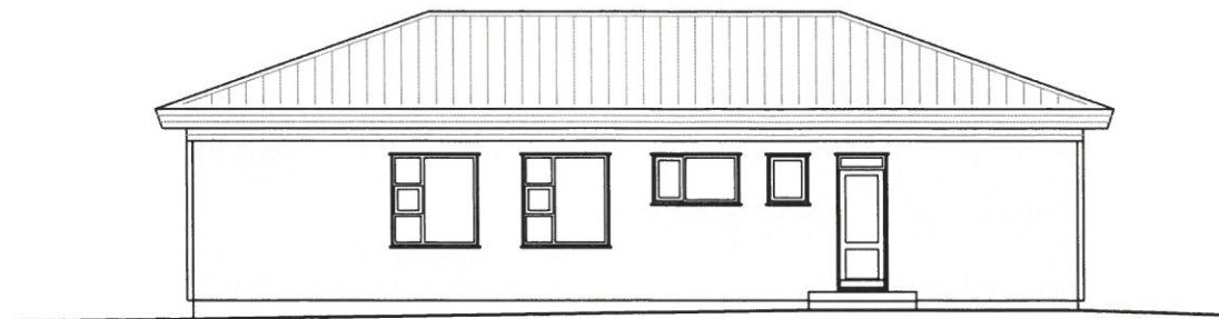
ÚTLIT NORÐUR 1:100
