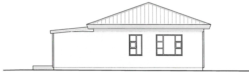
ÚTLIT AUSTUR 1:100
