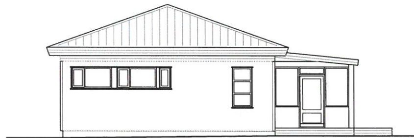
ÚTLIT VESTUR 1:100
