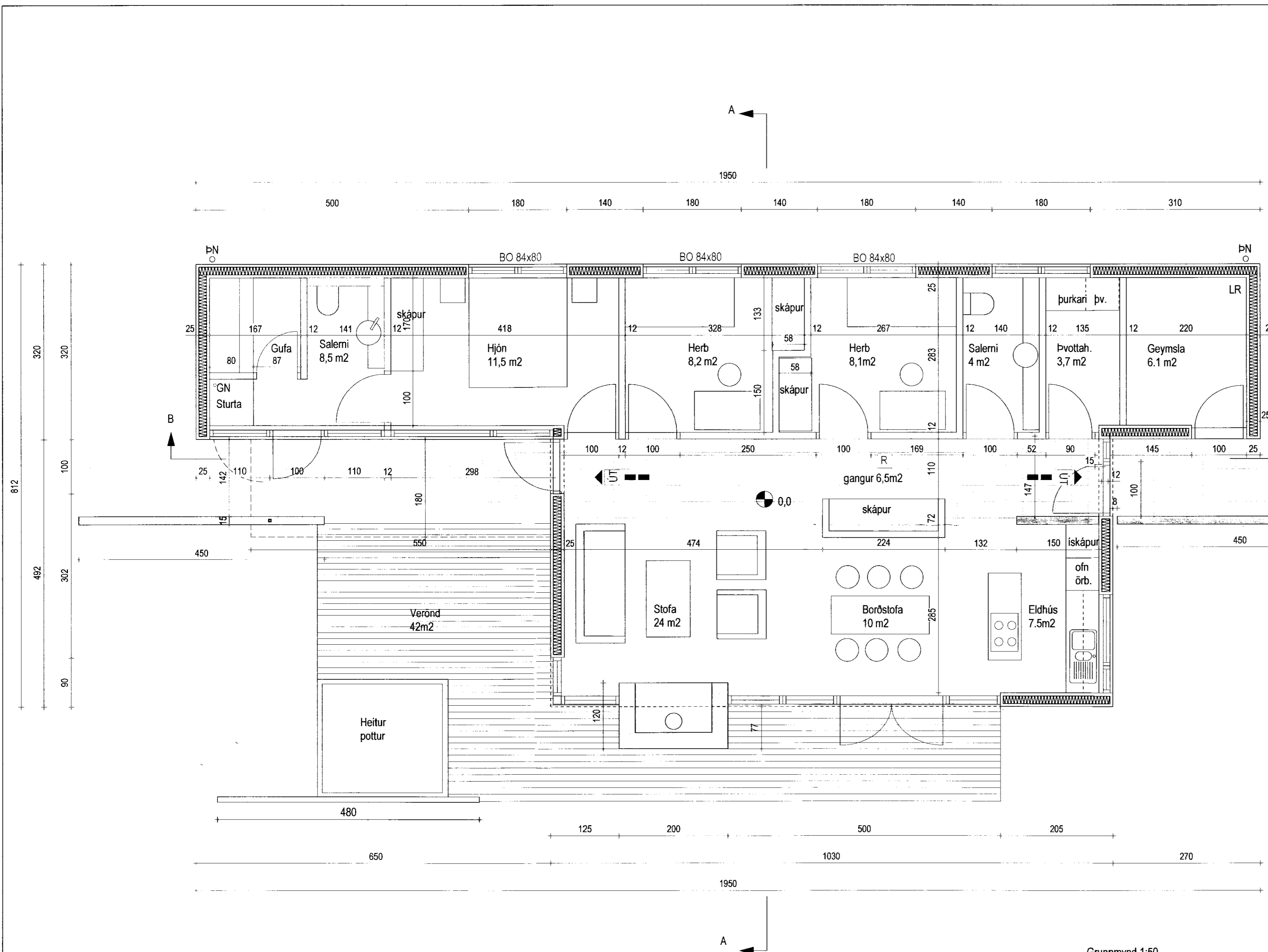
Grunnmynd 1:50
