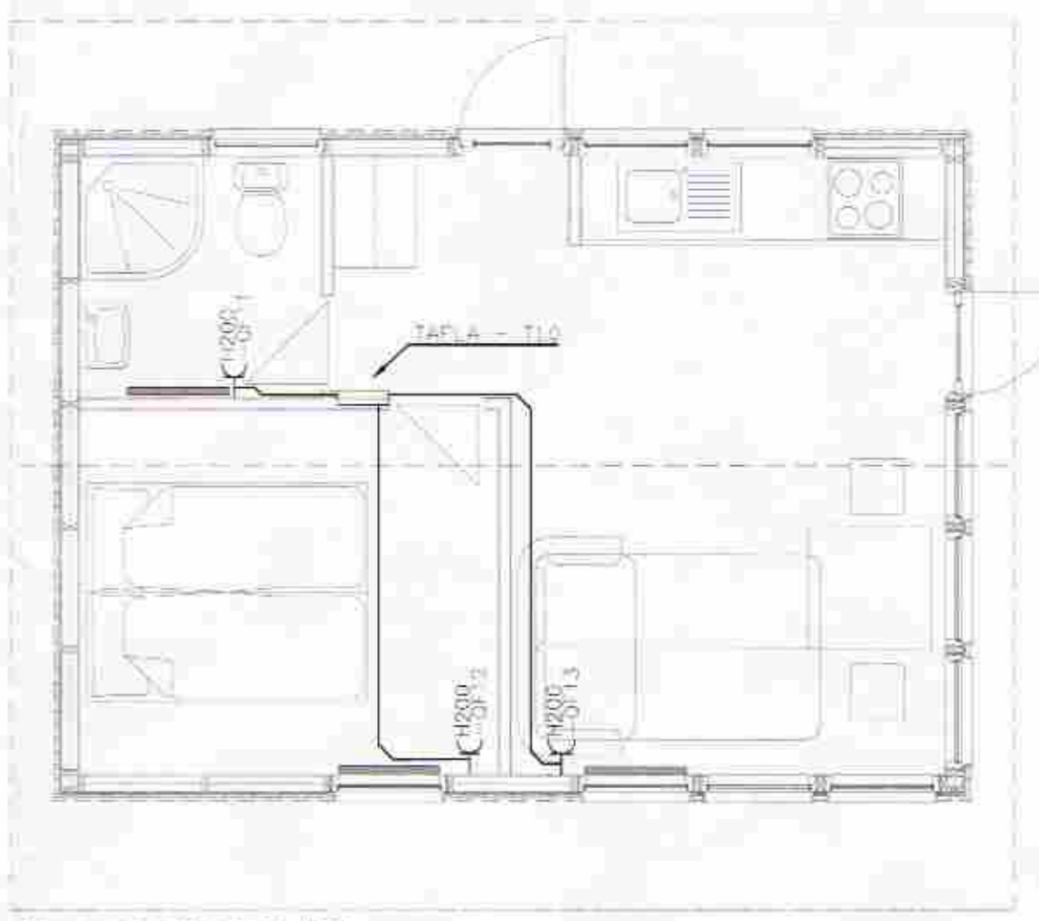
GRUNNMYND HITALÖGN MKV:1:50
