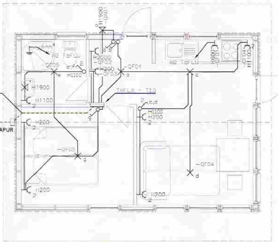
GRUNNMYND LJÓSA OG TENGLALÖGN MKV:1:50
