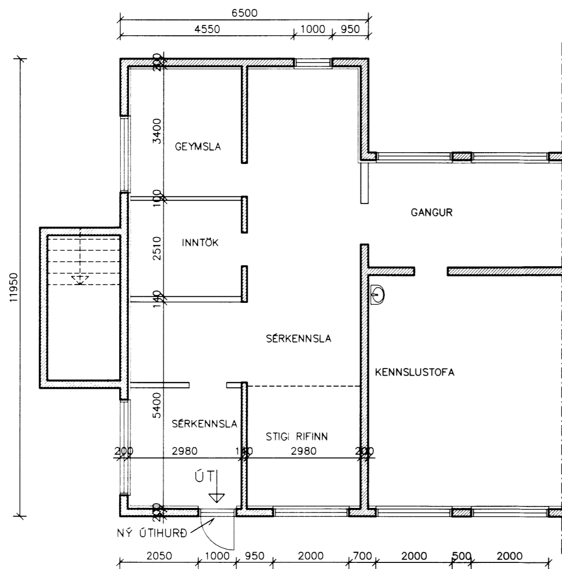
GRUNNMYND 1. HÆÐ MKV.1:100
