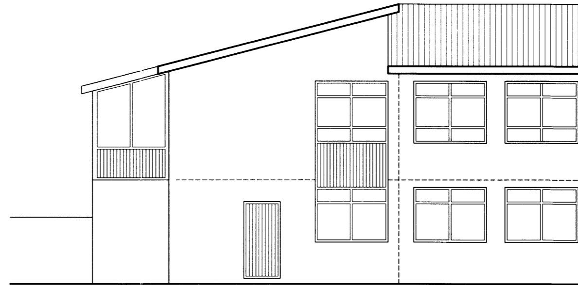
NORÐ-VESTUR MKV.1:100
