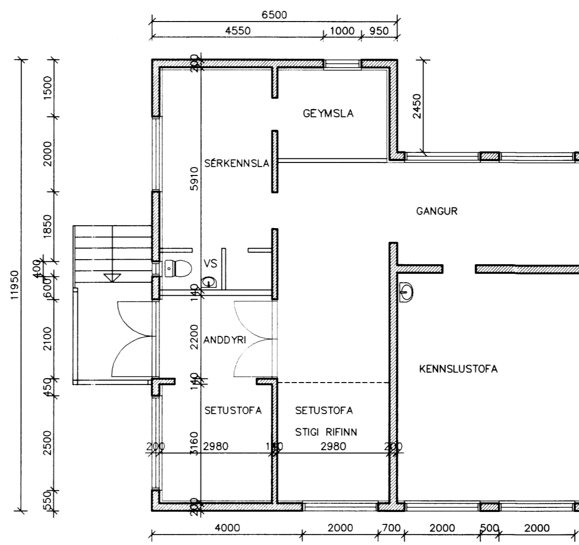
GRUNNMYND 2. HÆÐ MKV.1:100
