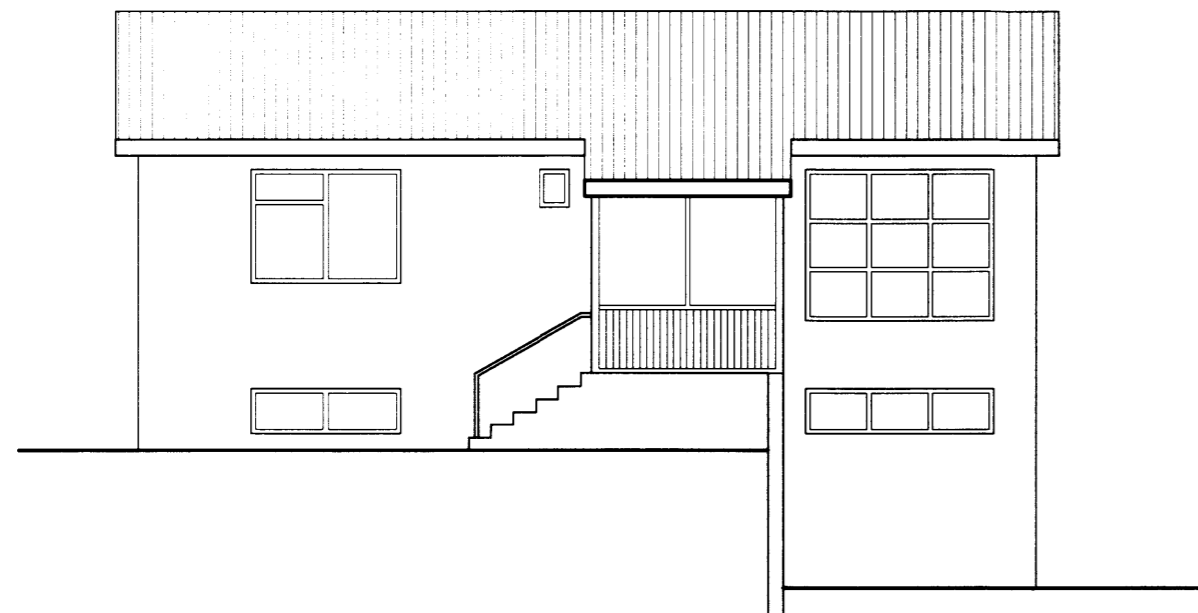
NORÐ-AUSTUR MKV.1:100
