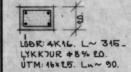
A-A 1:20
