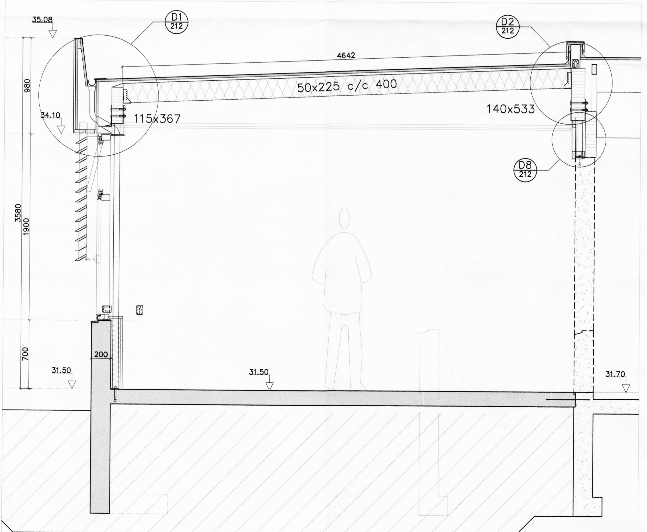
A Snið 1:20
