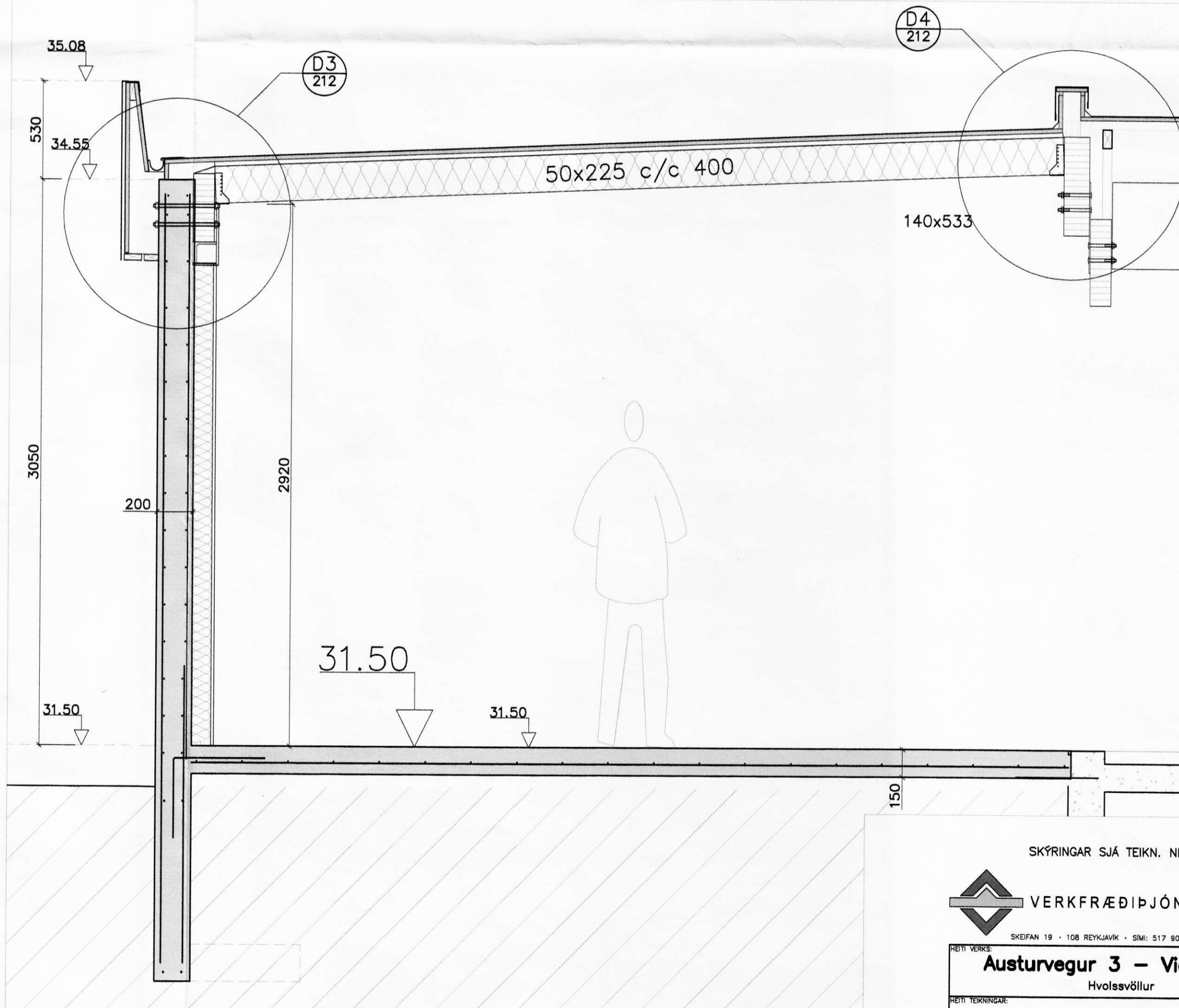
B Snið 1:20
