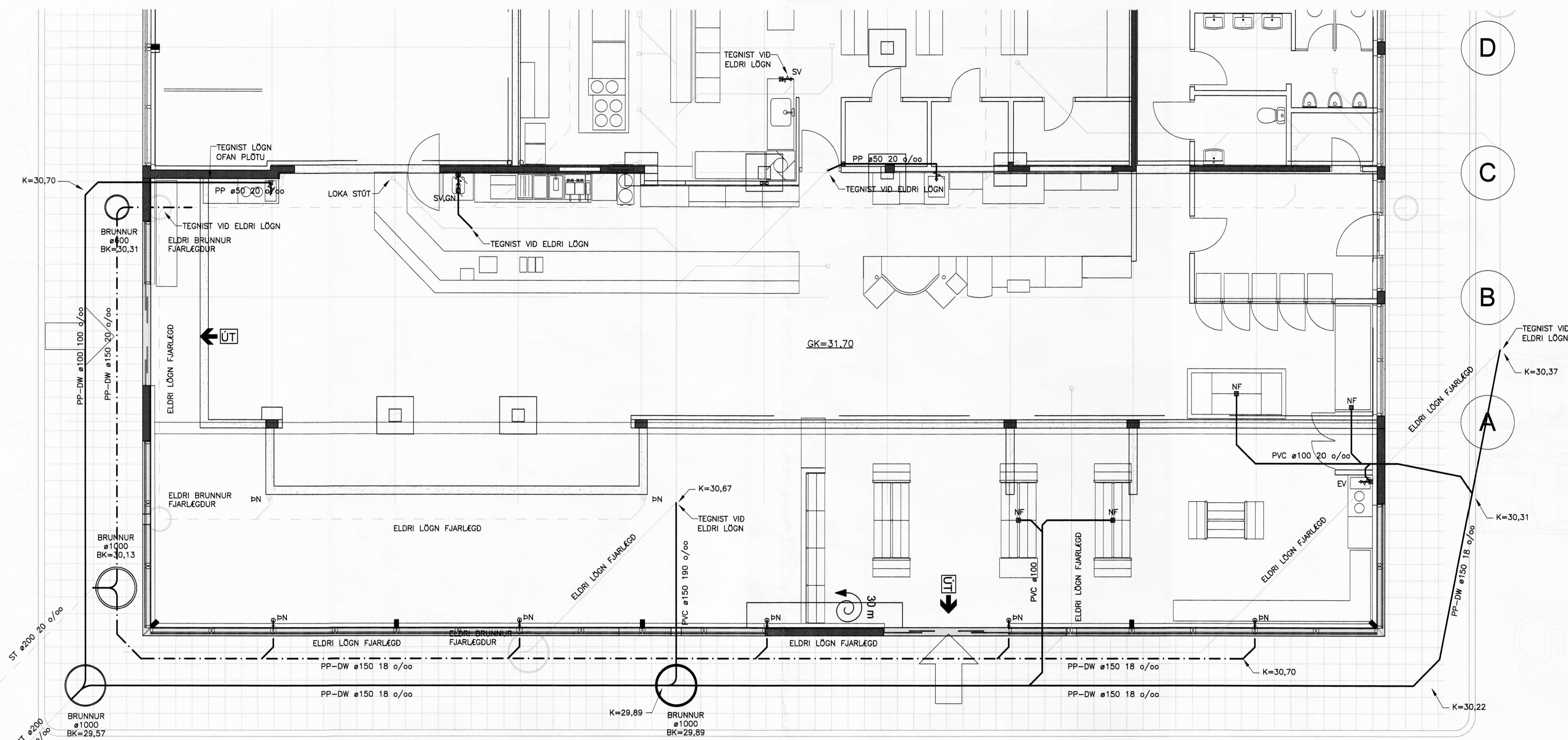
Grunnlagir. 1:50
