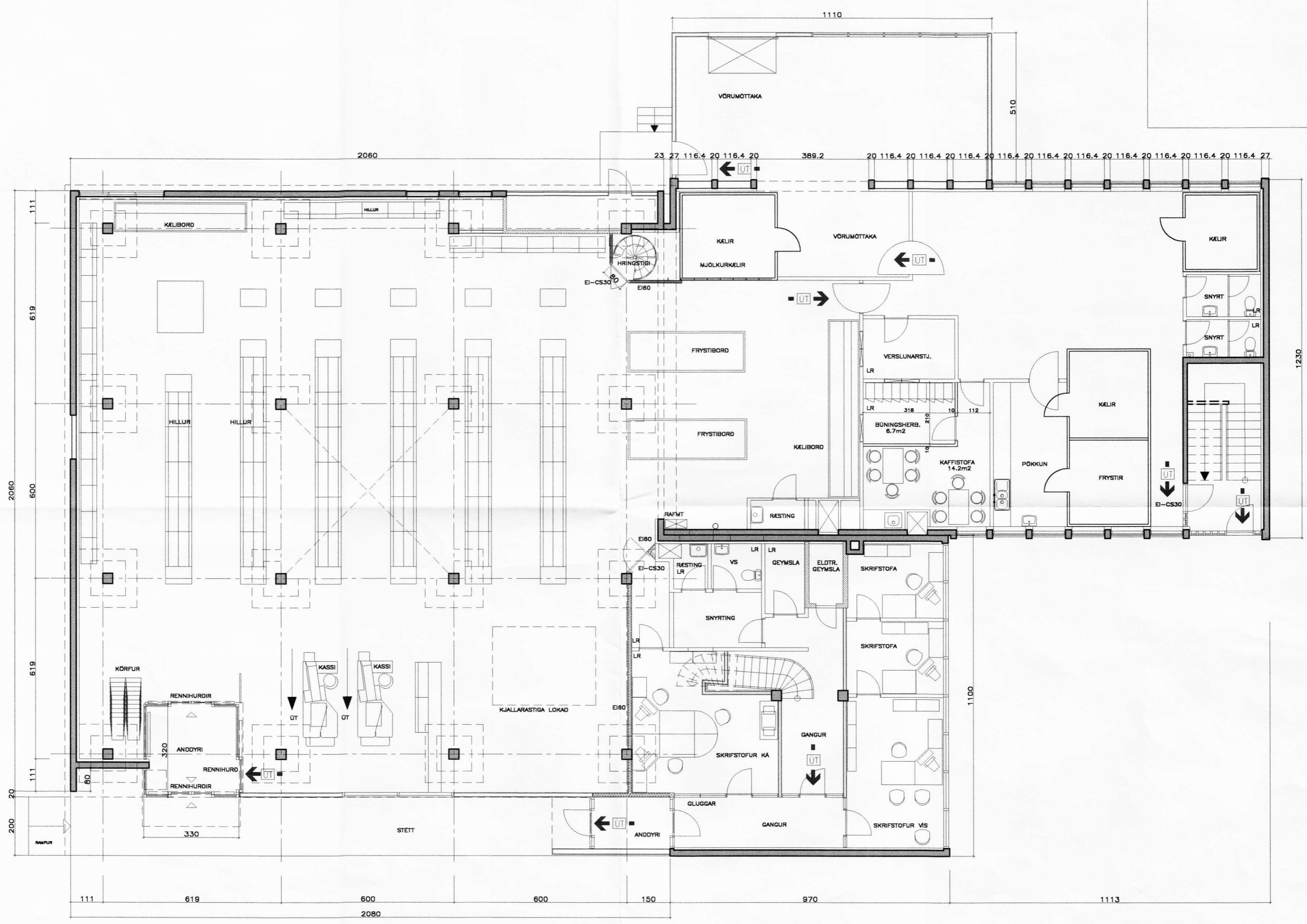
GRUNNMYND 1. HÆÐ
