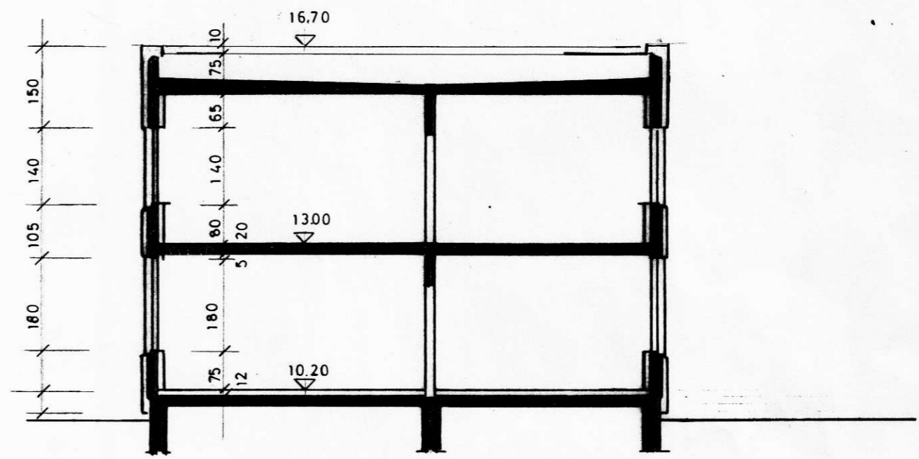
skurður A A
