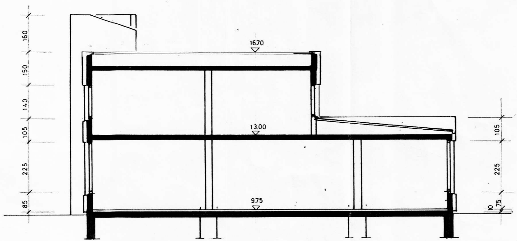
skurður B B
