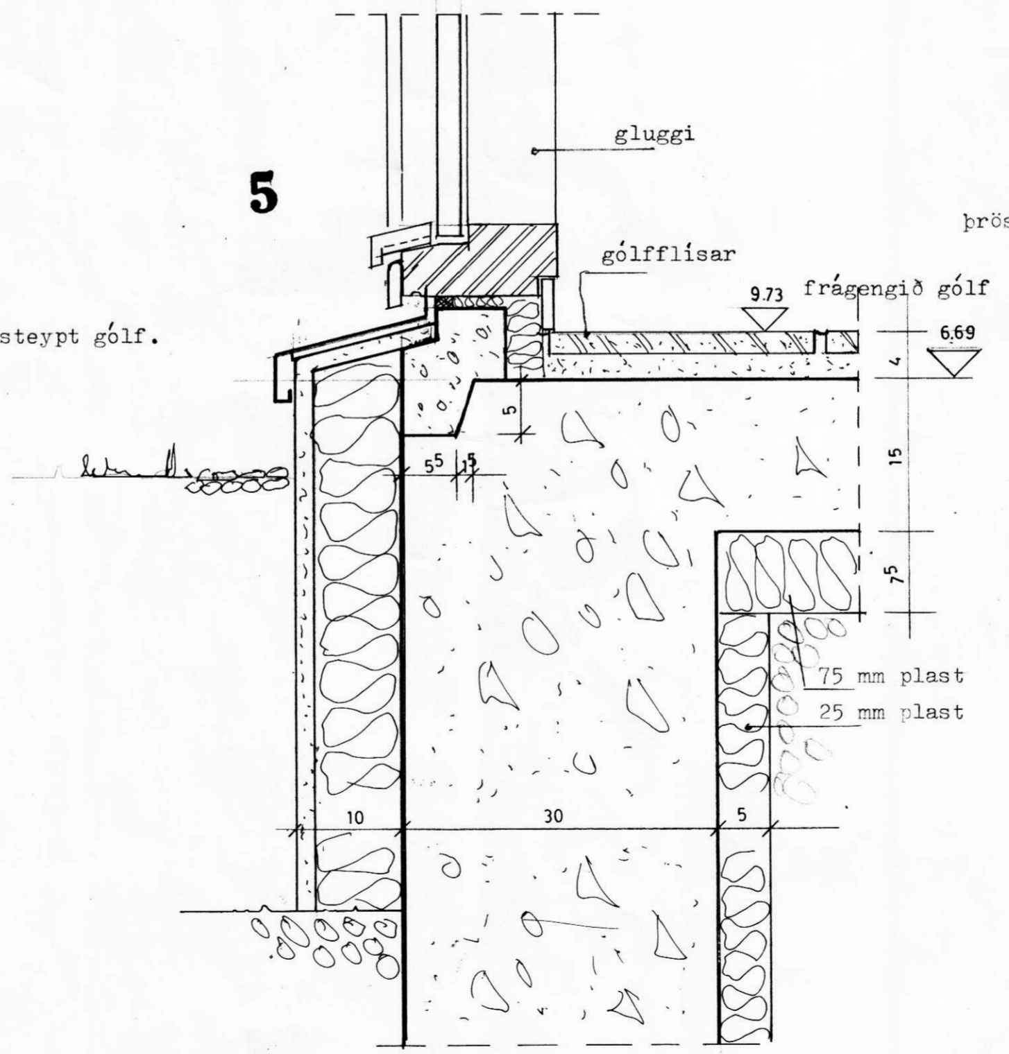
lóðréttur skurður
