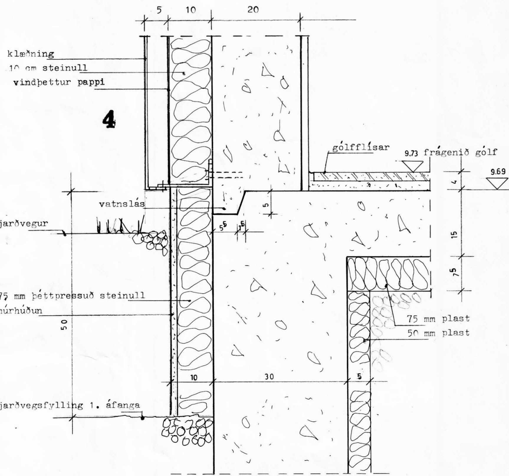
lóðréttur skurður
