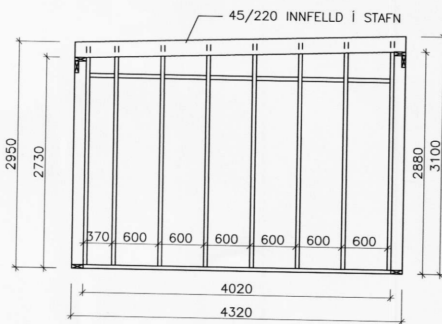
VEGGUR 4 1:50
