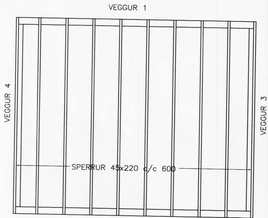
VEGGUR 2 ÞAK 1:50
