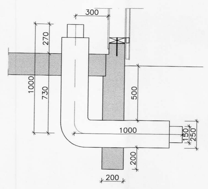
SNID Mkv: 1:20
