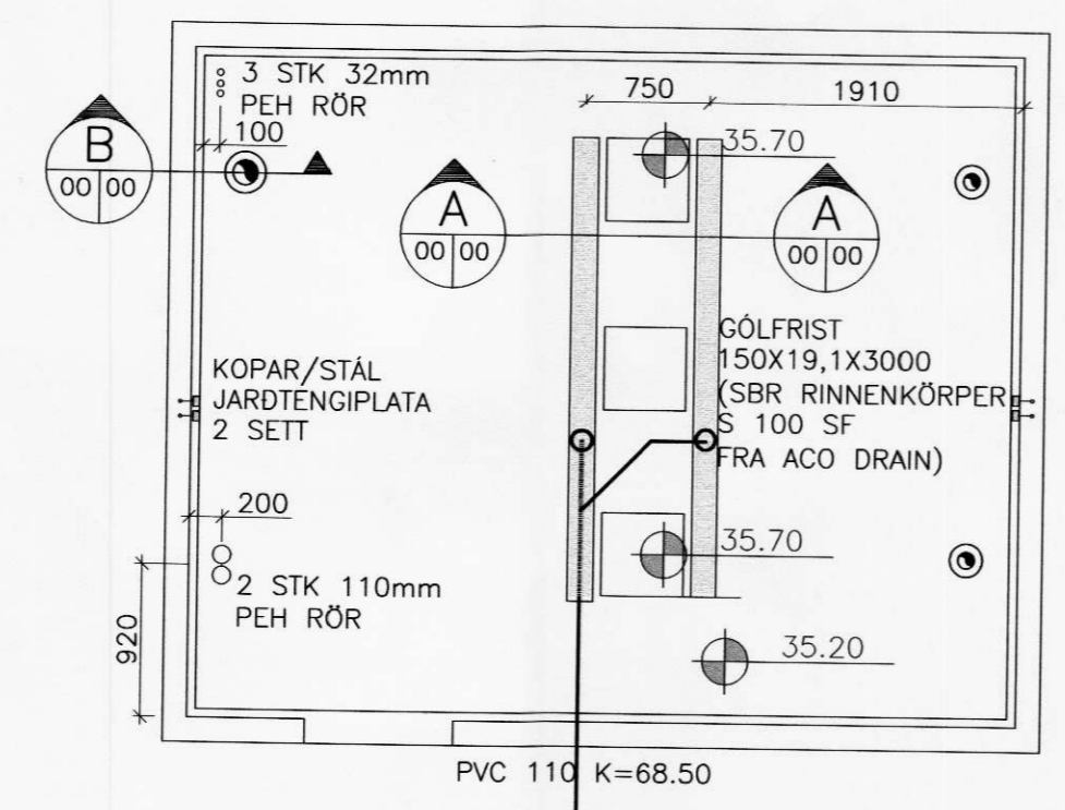
FRÁRENNSLISLAGNIR GRUNNMYND 1:50
