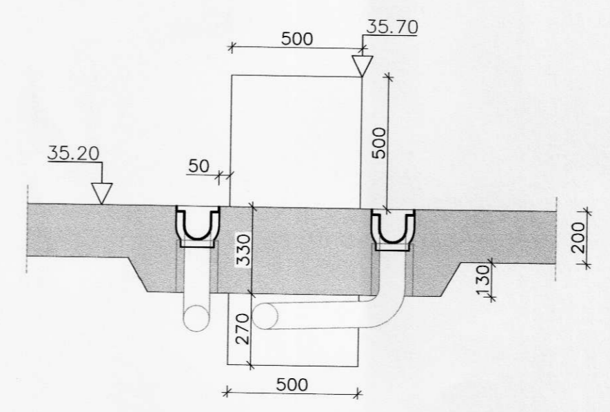
SNID Mkv: 1:20
