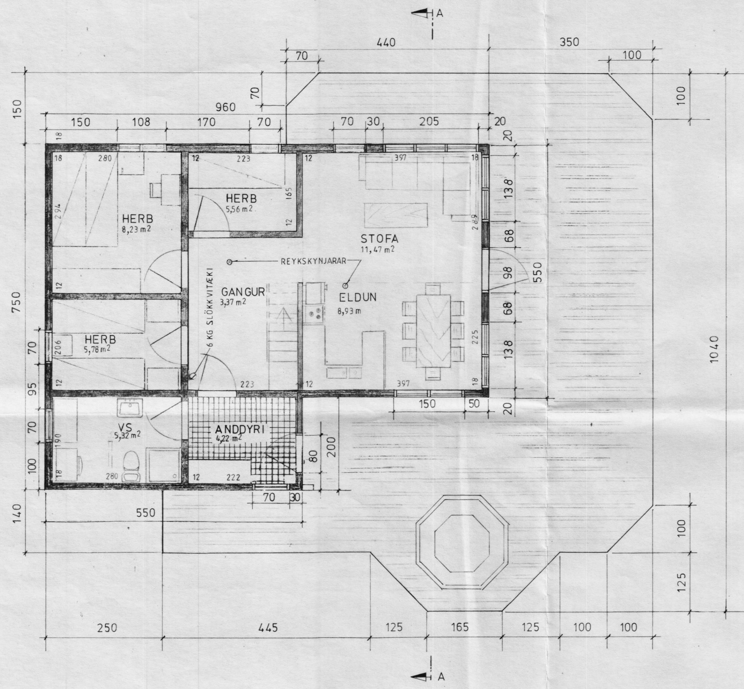
GRUNNMYND M = 1:50
