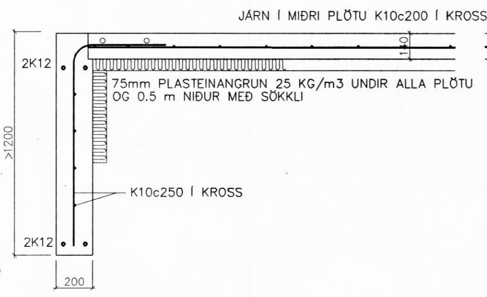
A-A 1:20
