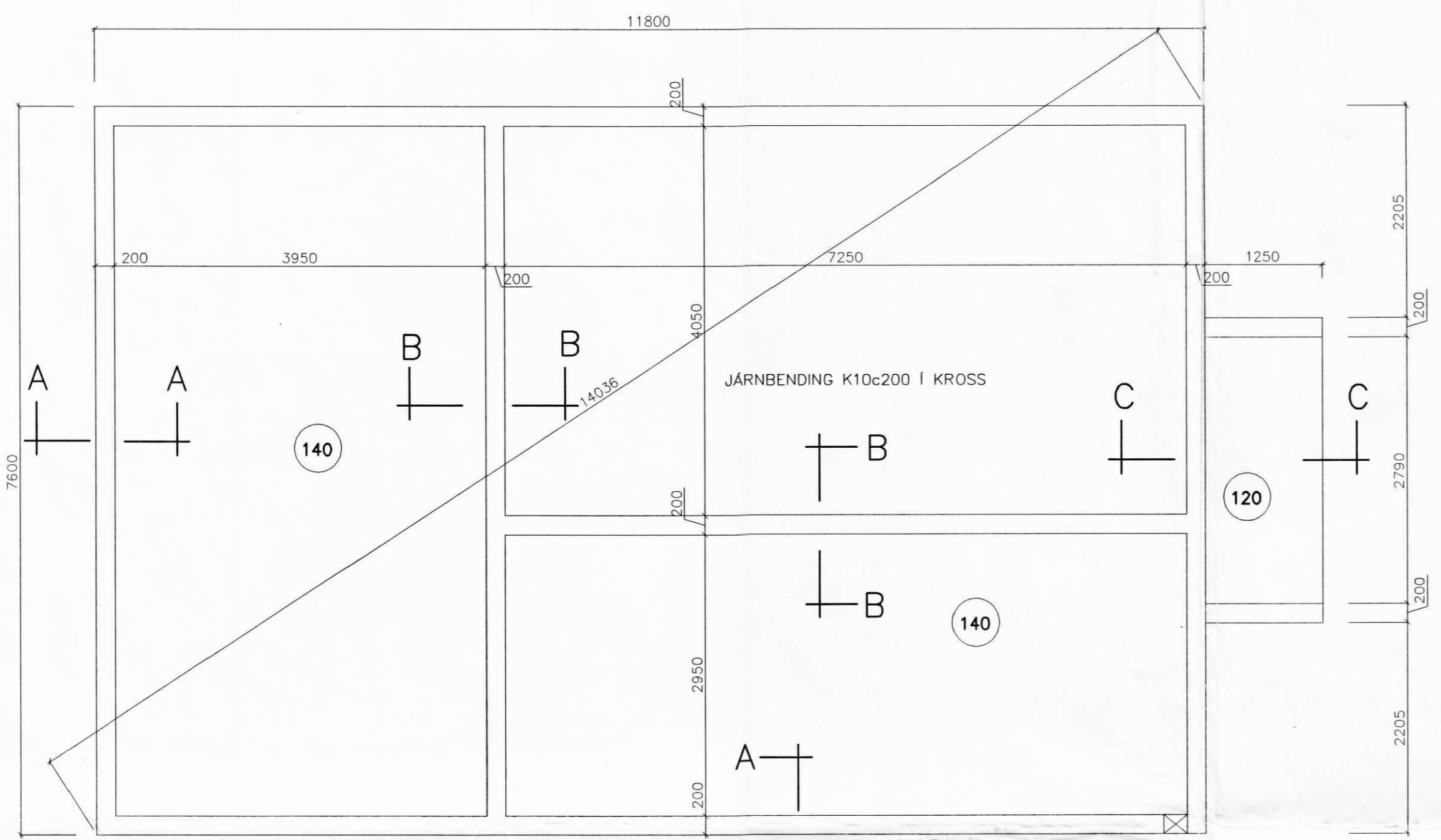
GRUNNMYND 1:50
