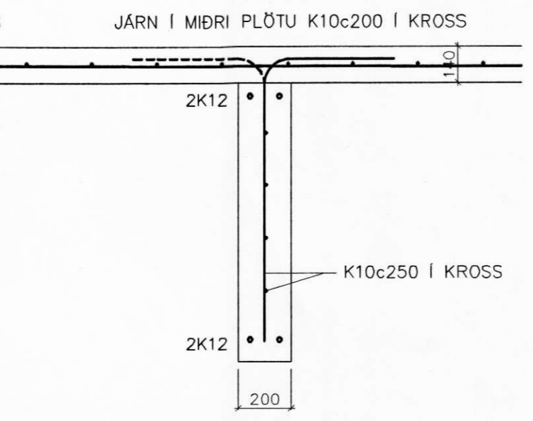
D-D 1:20
