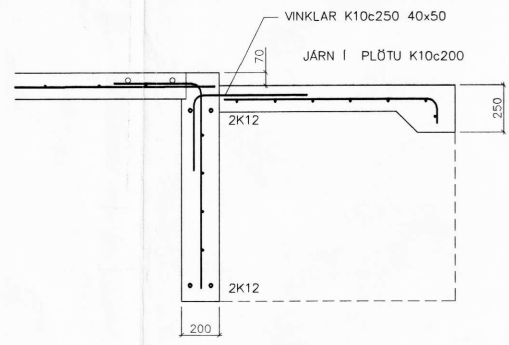
C-C 1:20
