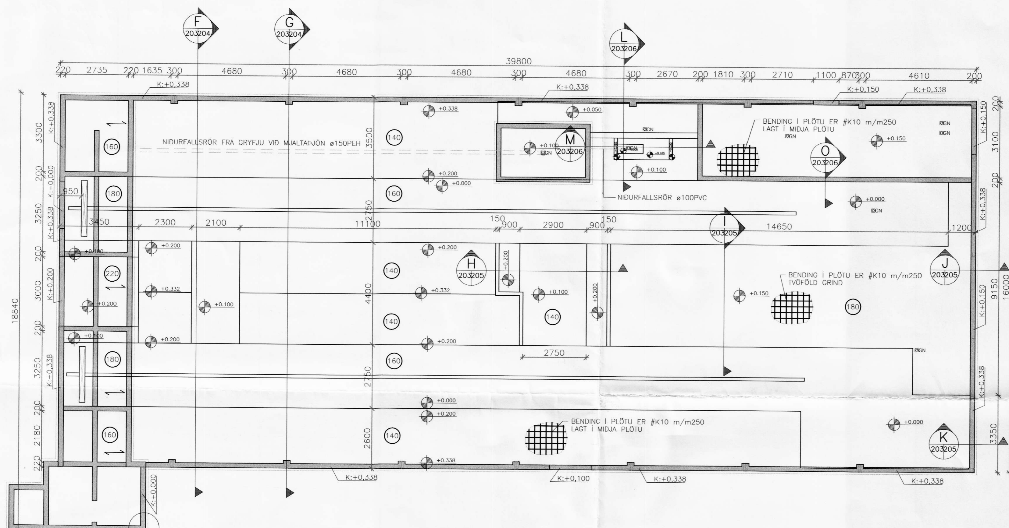
N 203206 GRUNNMYND 1:100
