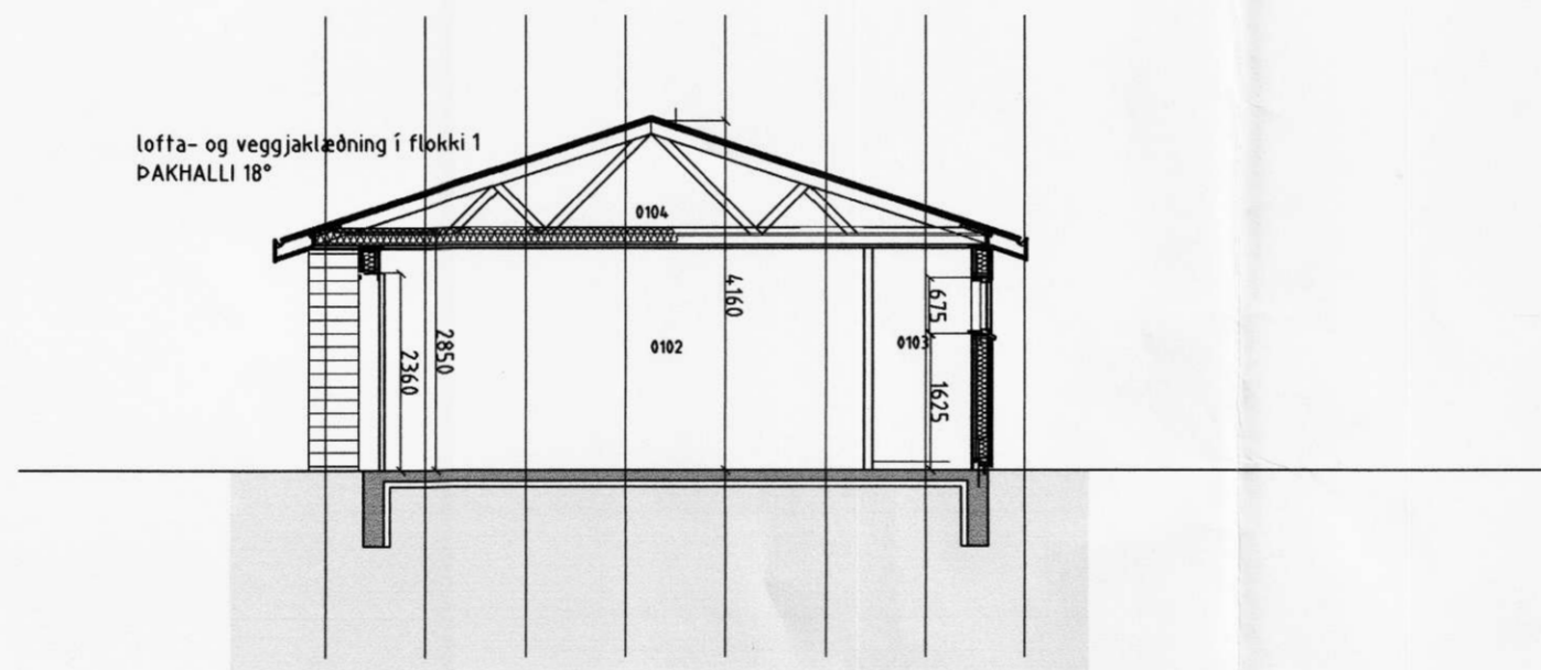
SNEIDMYND B-B
