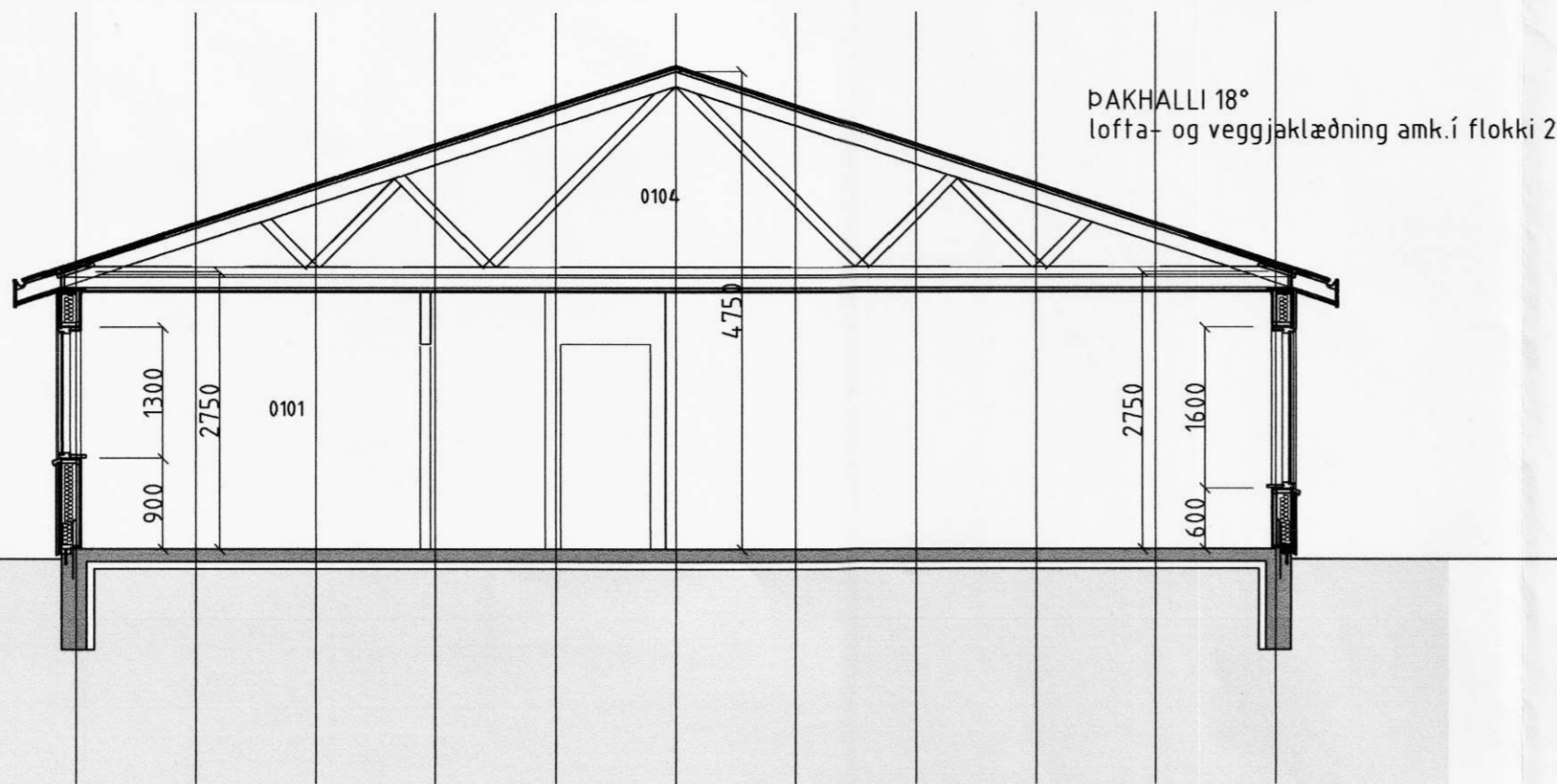
SNEIDMYND A-A
