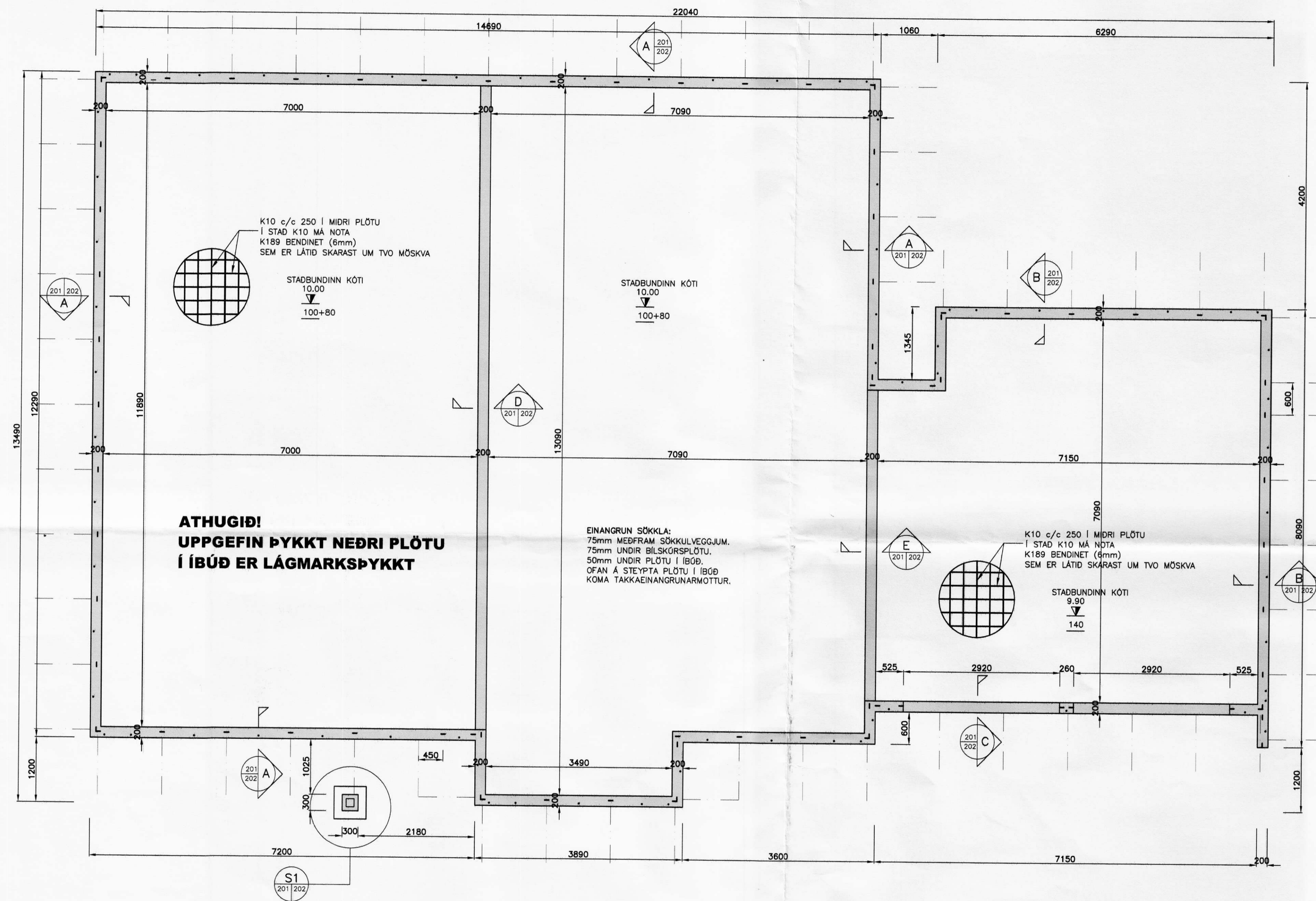
GRUNNMYND SÖKKULS MKV. 1:50
