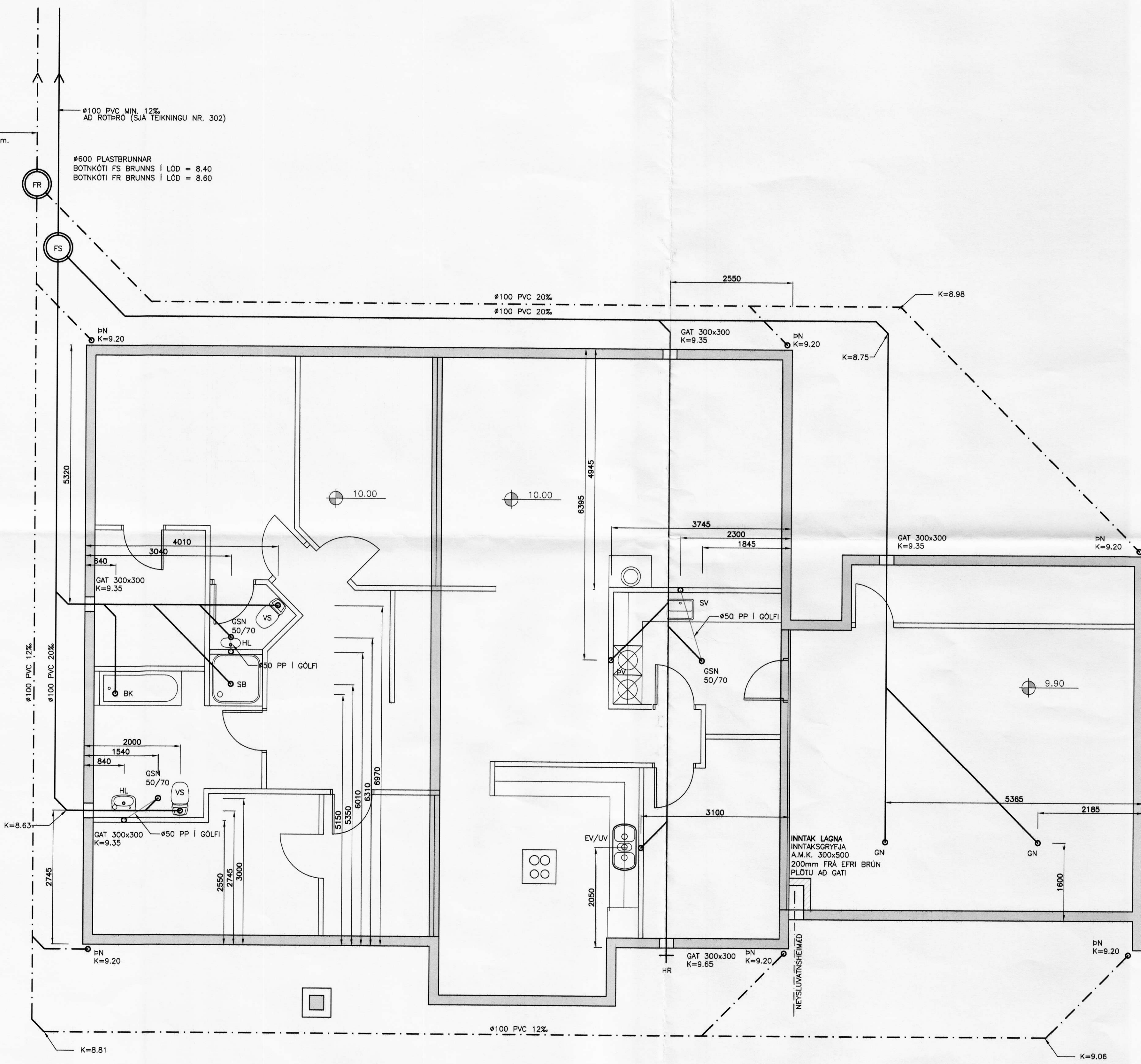
GRUNNMYND FRÁRENNISLAGNA MKV. 1:50
