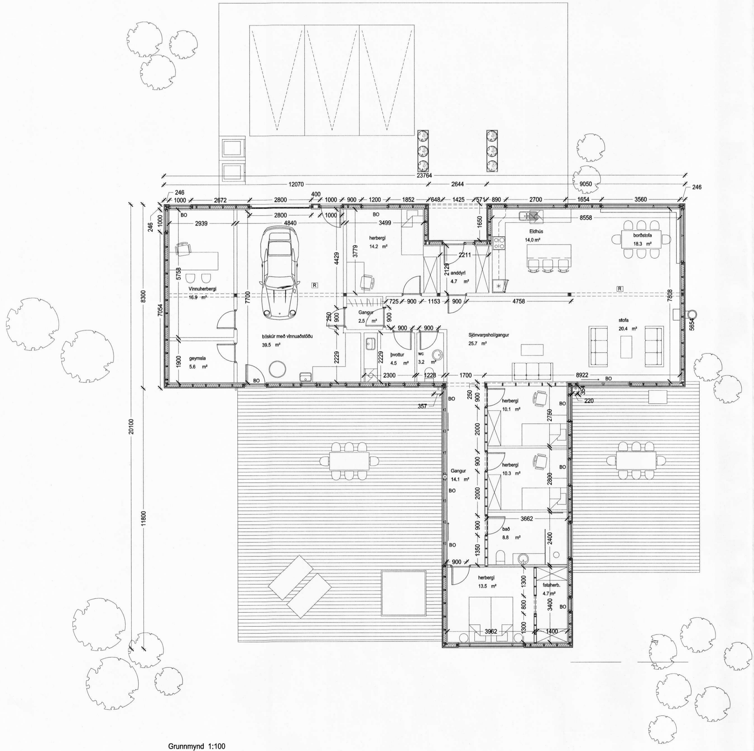
Grunnmynd 1:100
