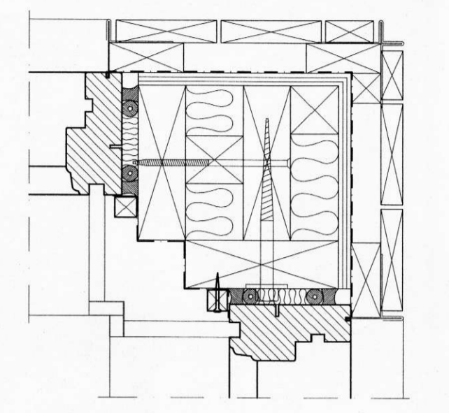
7 LÁRÉTT DEILI | ÚTHORN VÍÐ (99)3.01 STOFUGLUGG, TIMBURKLÆÐNING
