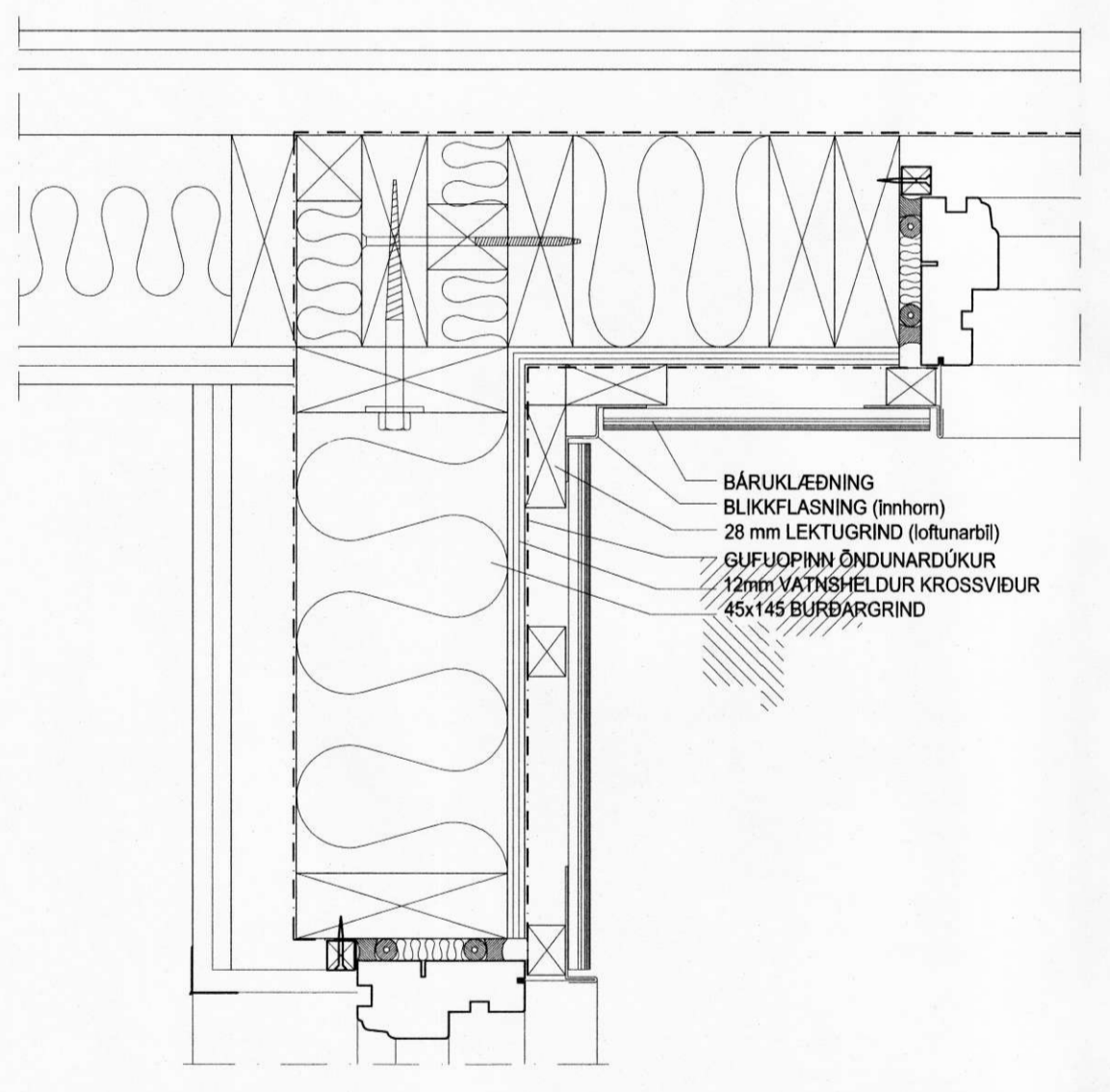
8 LÁRÉTT DEILI | INNHORN (99)3.01 BÁRUKLÆÐNINGAR VÍÐ HERBERGISÁLMU
