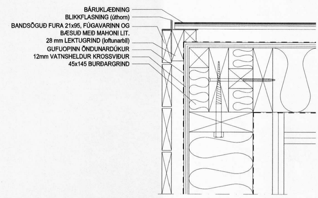
6 LÁRÉTT DEILI | ÚTHORN VÍÐ (99)3.01 ADALINNGANG, TIMBUR / BÁRUKL.
