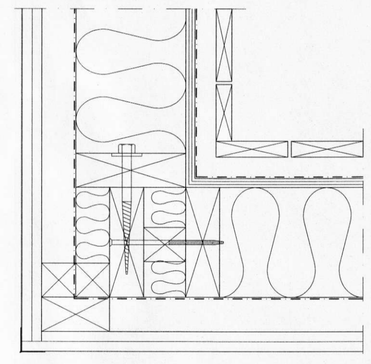
5 LÁRÉTT DEILI | INNHORN VÍÐ (99)3.01 ADALINNGANG
