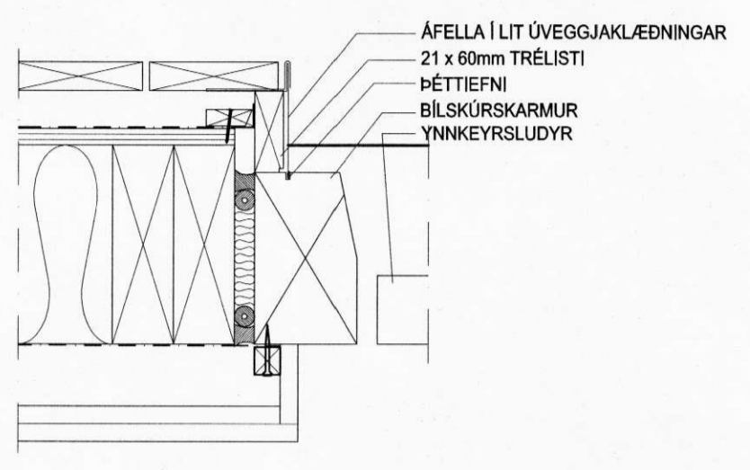
3 LÁRÉTT DEILI | (99)3.01 INNKEYRSLUÐYR | BÍLSKÚR
