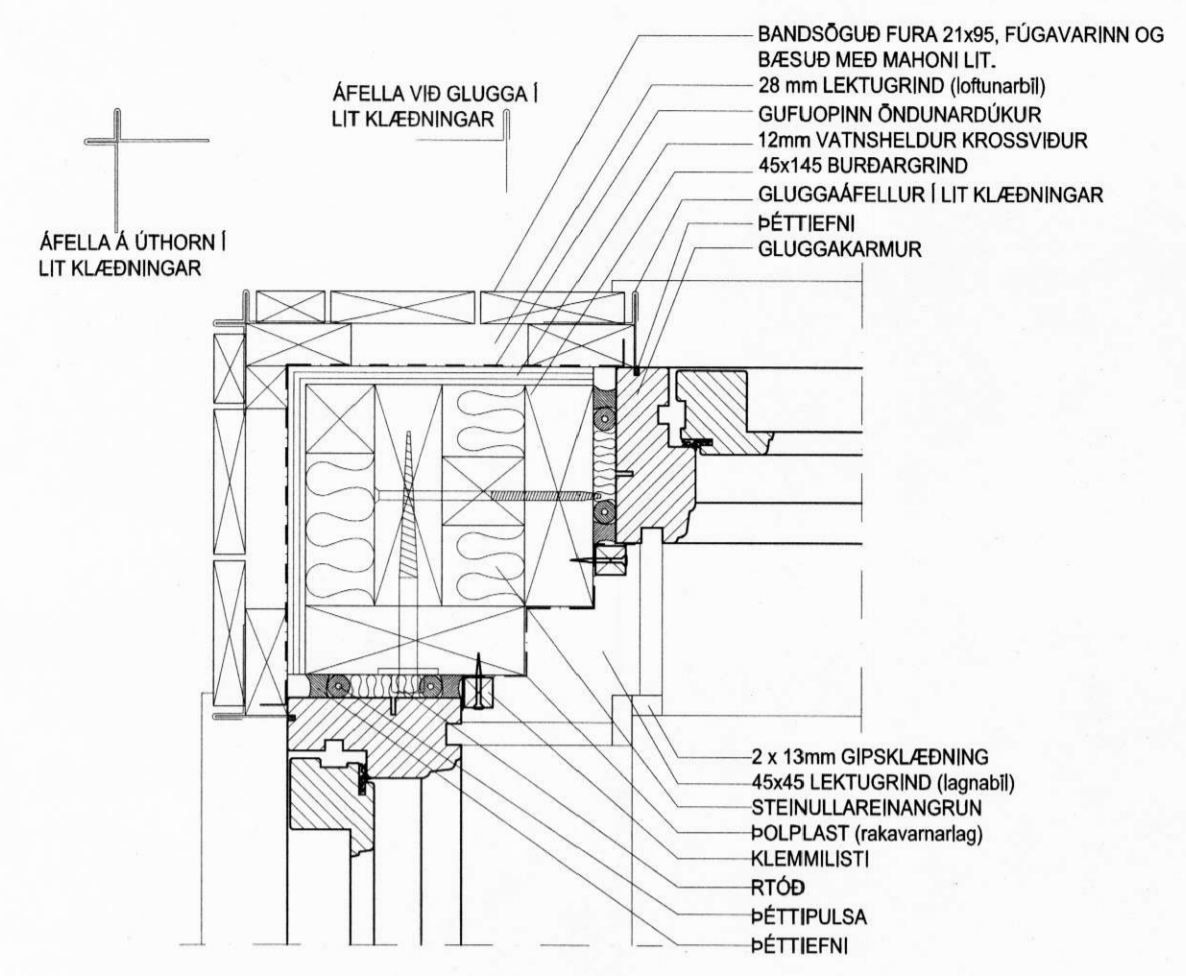
1 LÁRÉTT DEILI | ÚTHORN (99)3.01 VÍÐ GLUGGA OG TIMBURKLÆÐNINGU
