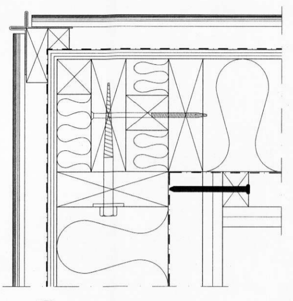
2 LÁRÉTT DEILI | ÚTHORN (99)5.01 OFAN VÍÐ GLUGGA, BÁRUKLÆÐNING
