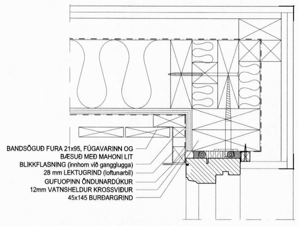
9 LÁRÉTT DEILI | INNHORN (99)3.01 Á HERBERGISGANGI
