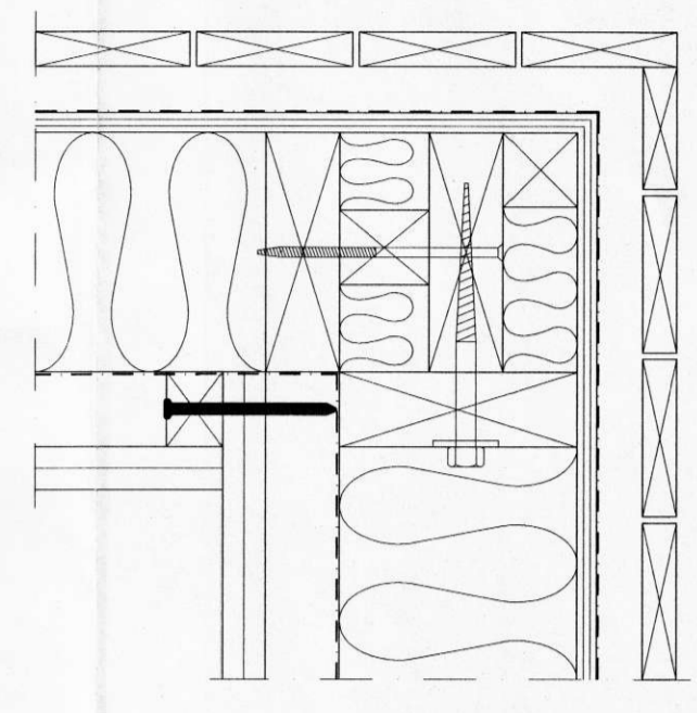
4 LÁRÉTT DEILI | ÚTHORN VÍÐ (99)3.01 ADALINNGANG, TIMBURKLÆÐNING
