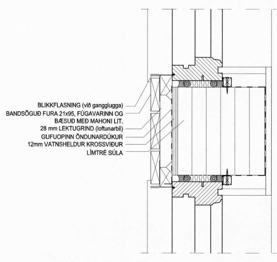
10 LÁRÉTT DEILI | BURÐARSÓLU (99)3.01 OG GLUGGA Á HERBERGISGANGI
