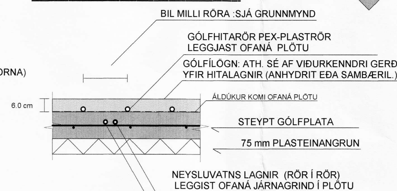
NEDRI HÆÐ: SNIÐ Í PLÖTU MKV. 1:10
