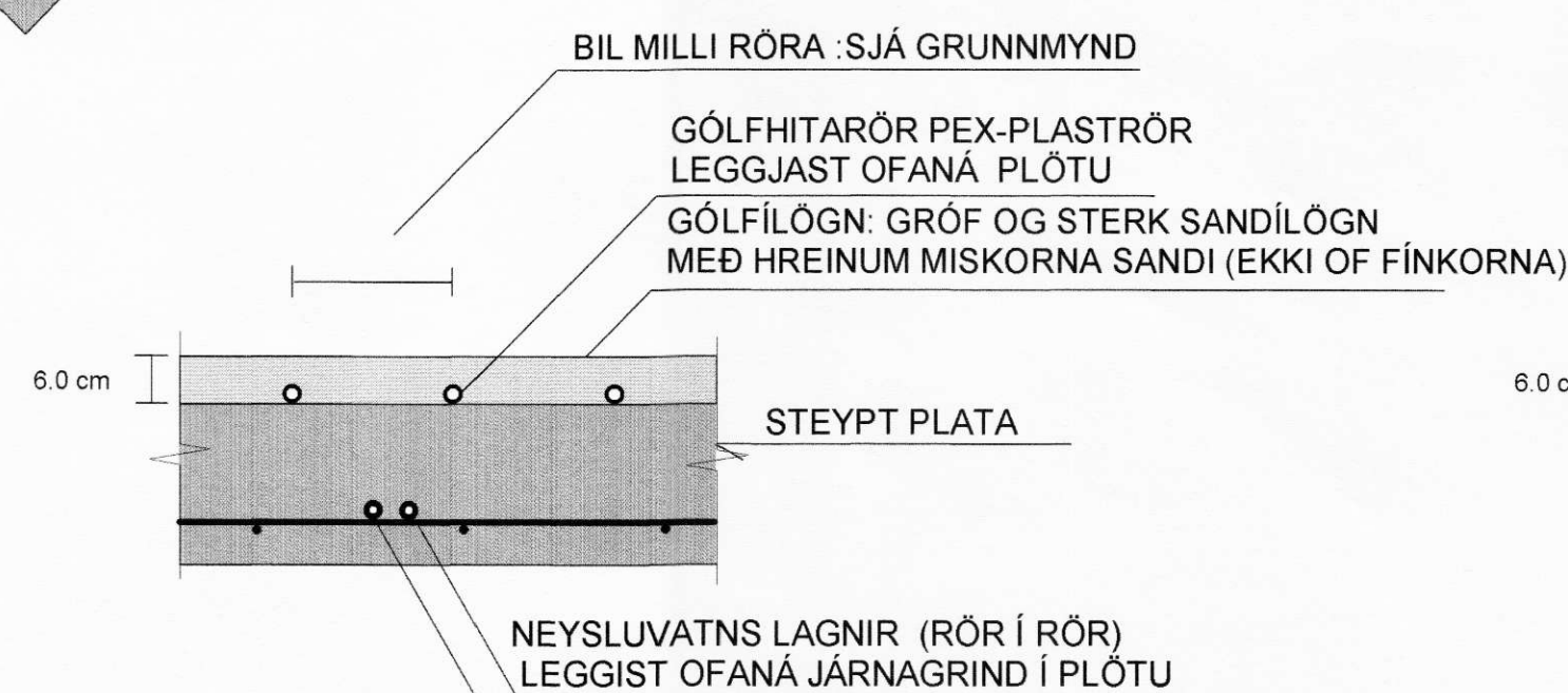
EFRI HÆÐ: SNIÐ Í PLÖTU - BÍLSKÚR MKV. 1:10
