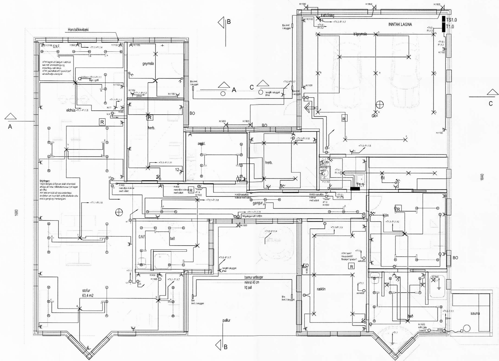
GRUNNMYND 1:50
