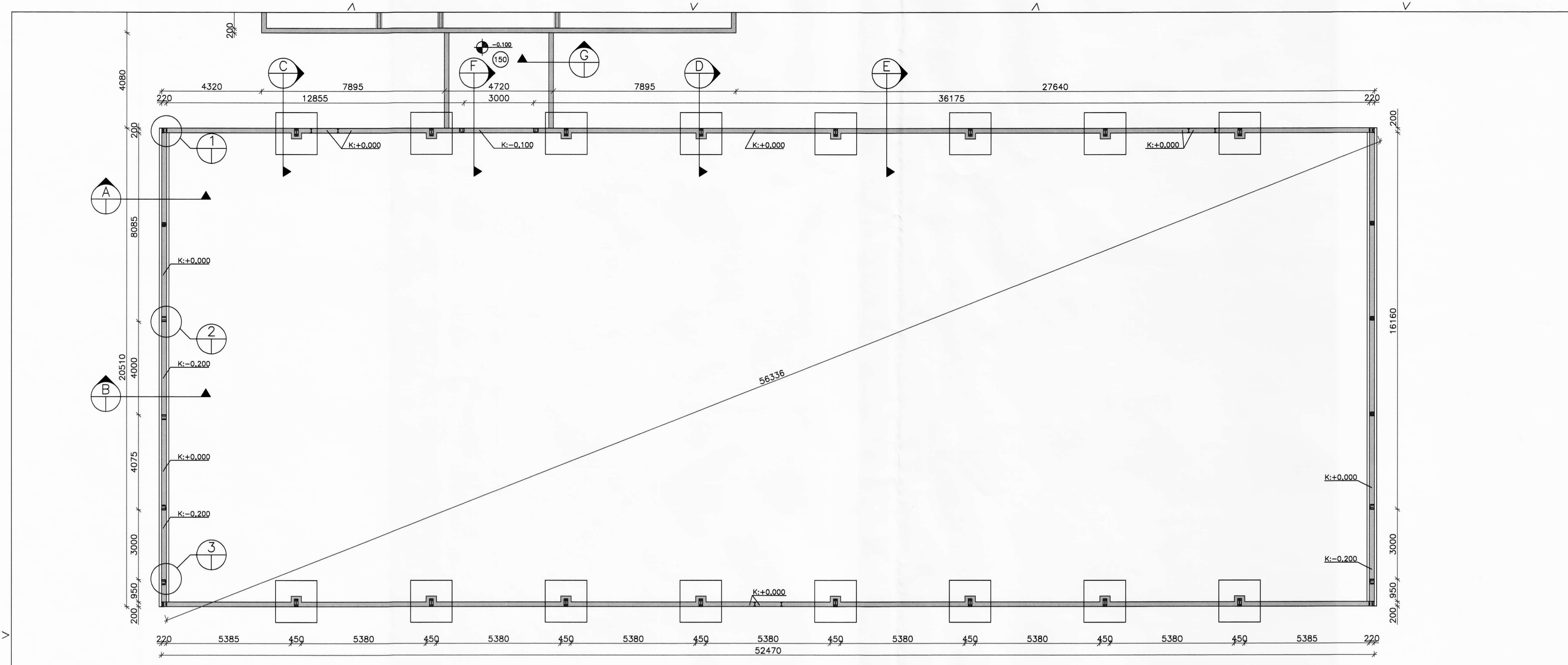
GRUNNMYND 1:100
