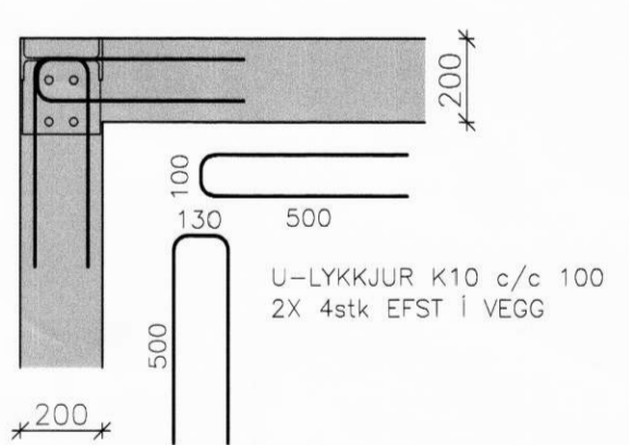
DEILI 4 Mkv: 1:20
