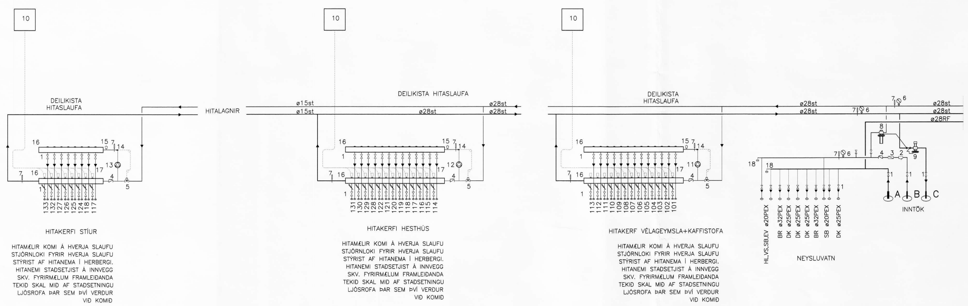
KERFISMYND STJÓRNÞUNADAR HITÁ- OG NEYSLUVATNSLAGNA
