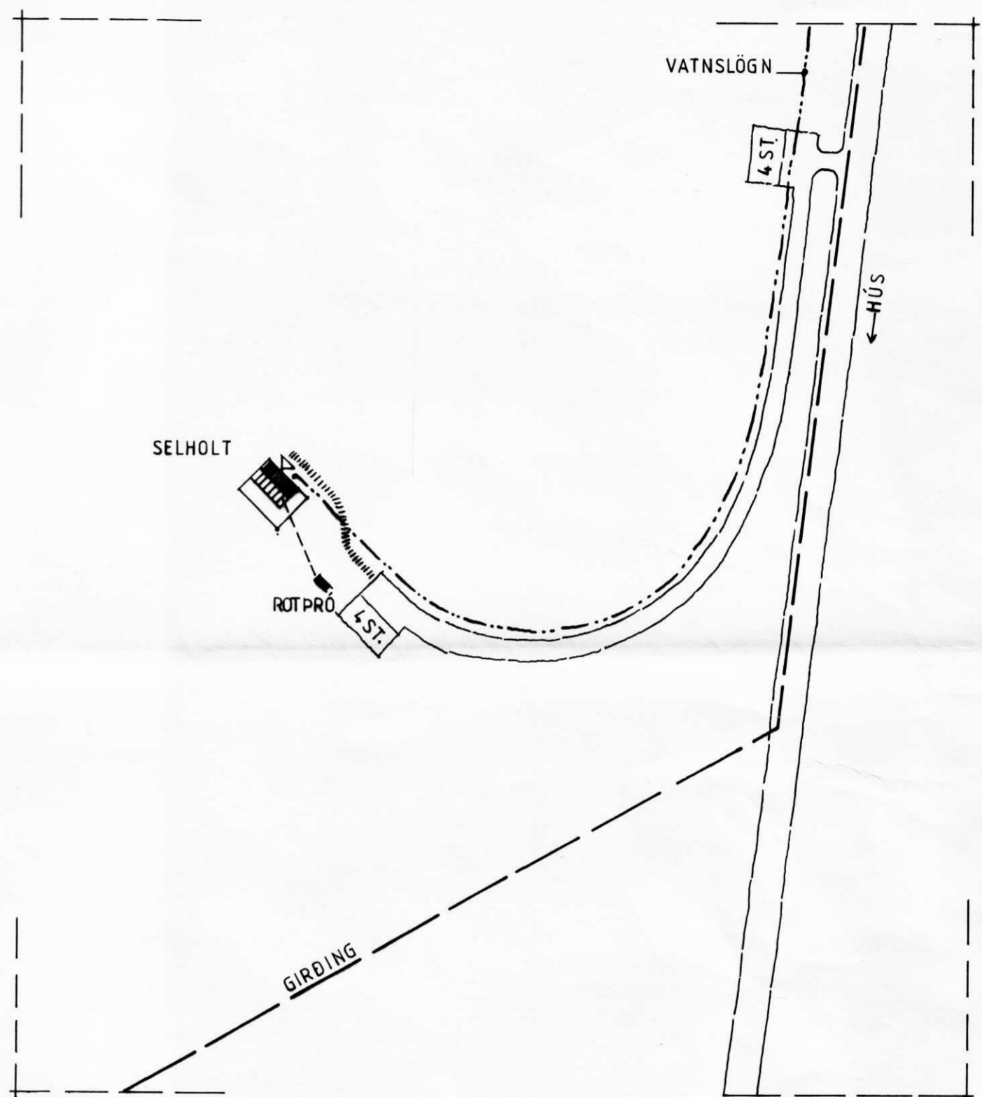
AFSTÖÐUMYND 1:1000
