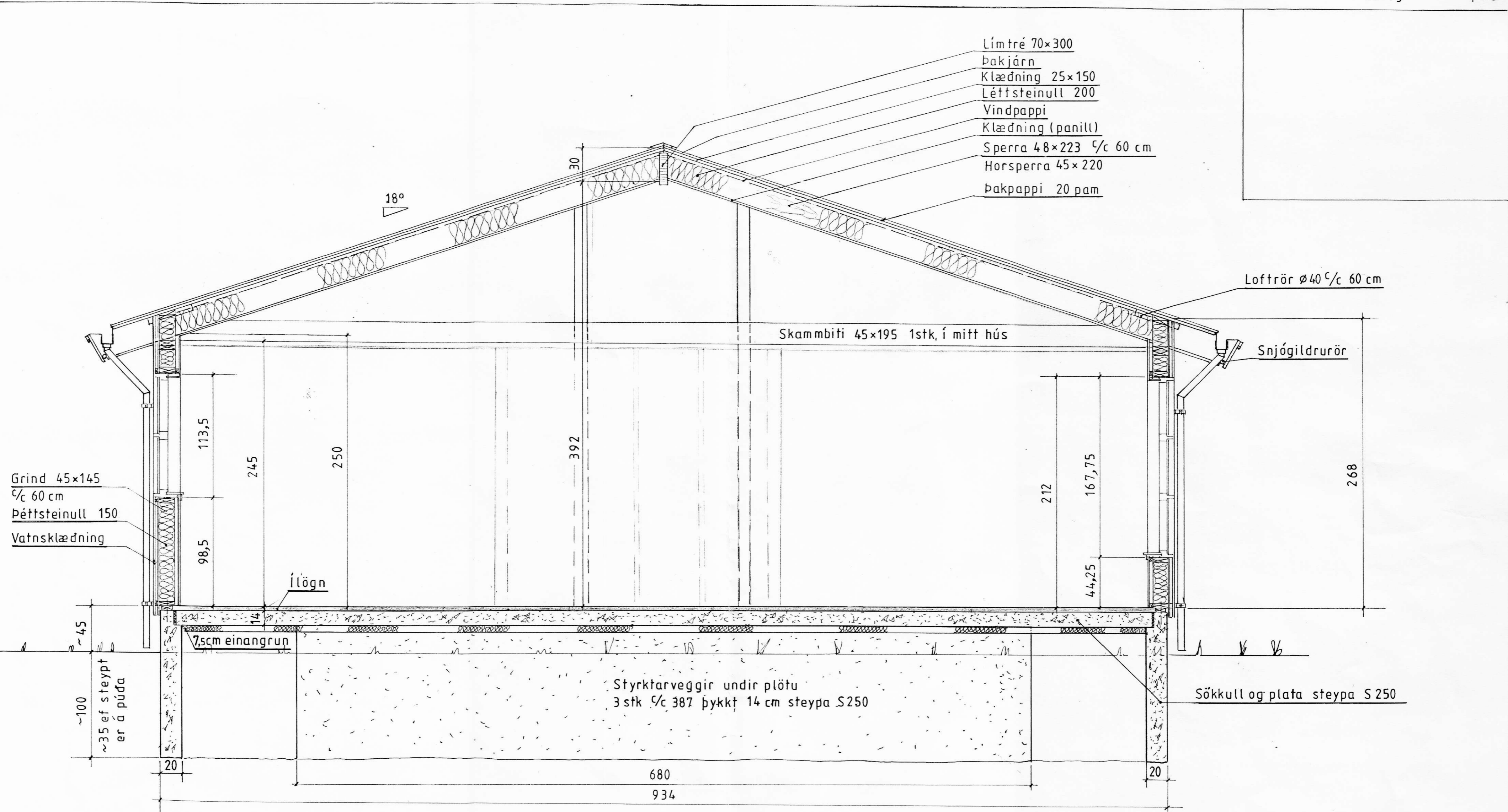
Snið A-A
