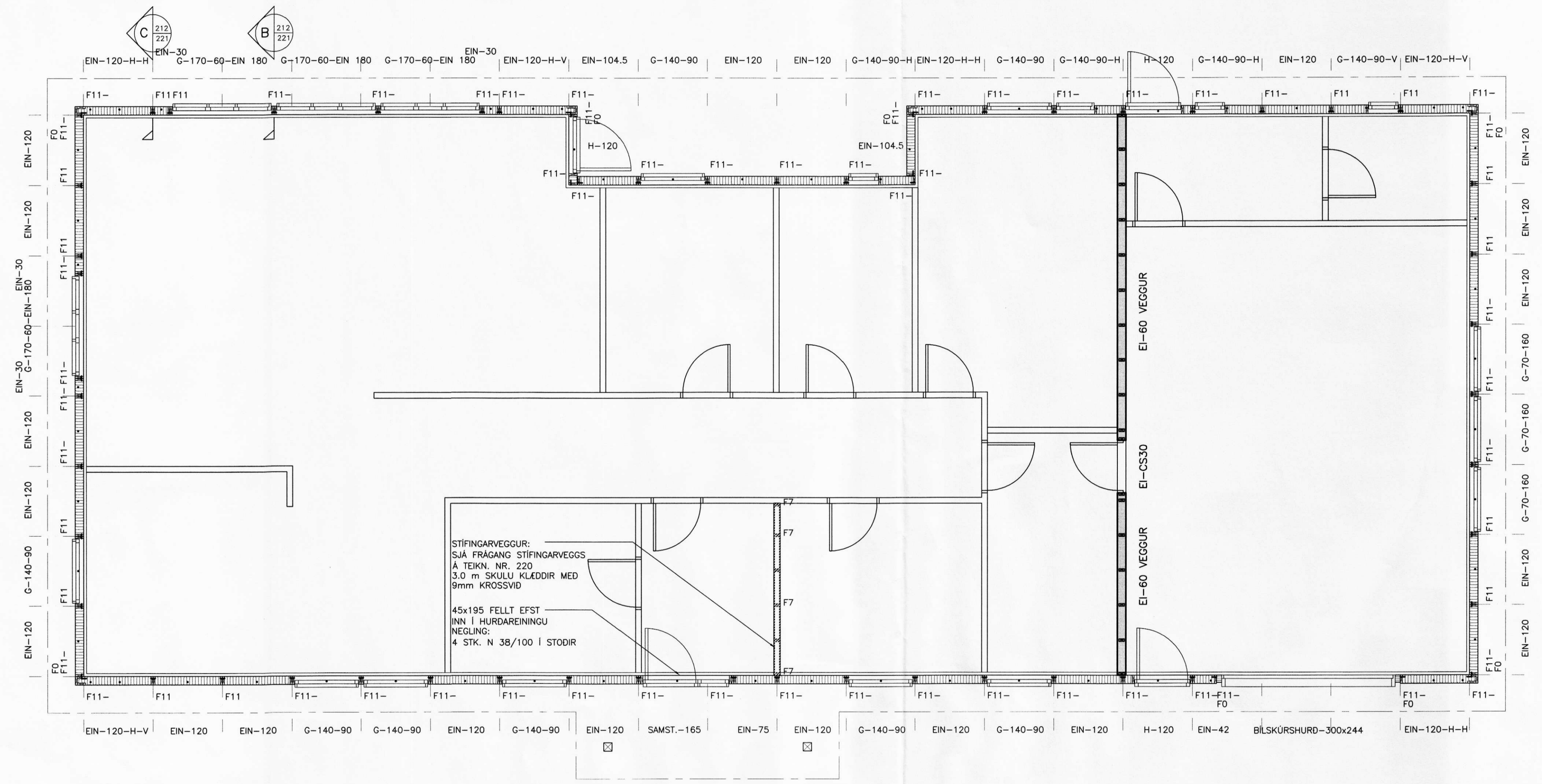
VEGGJAPLAN MKV. 1:50
