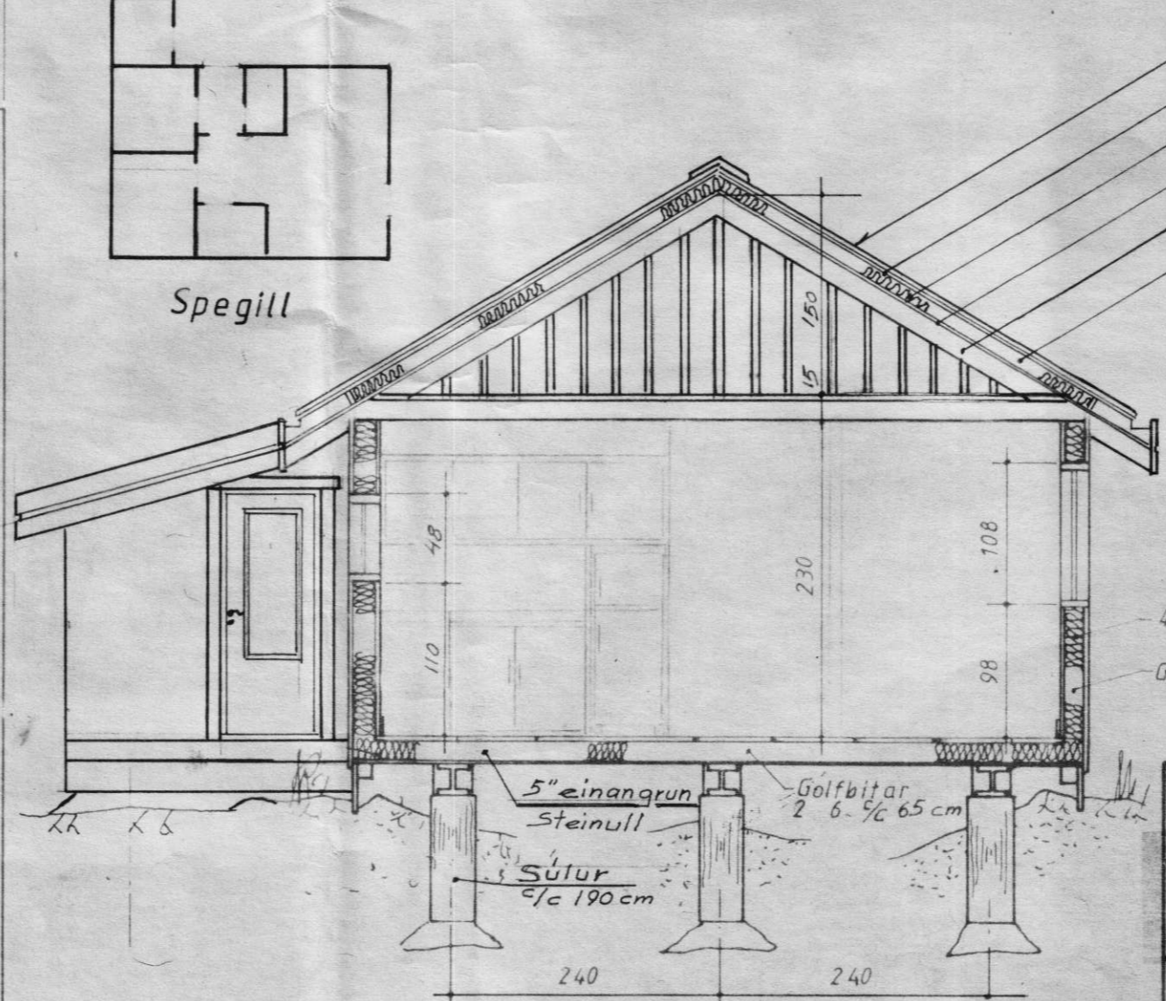
Snid A-A
