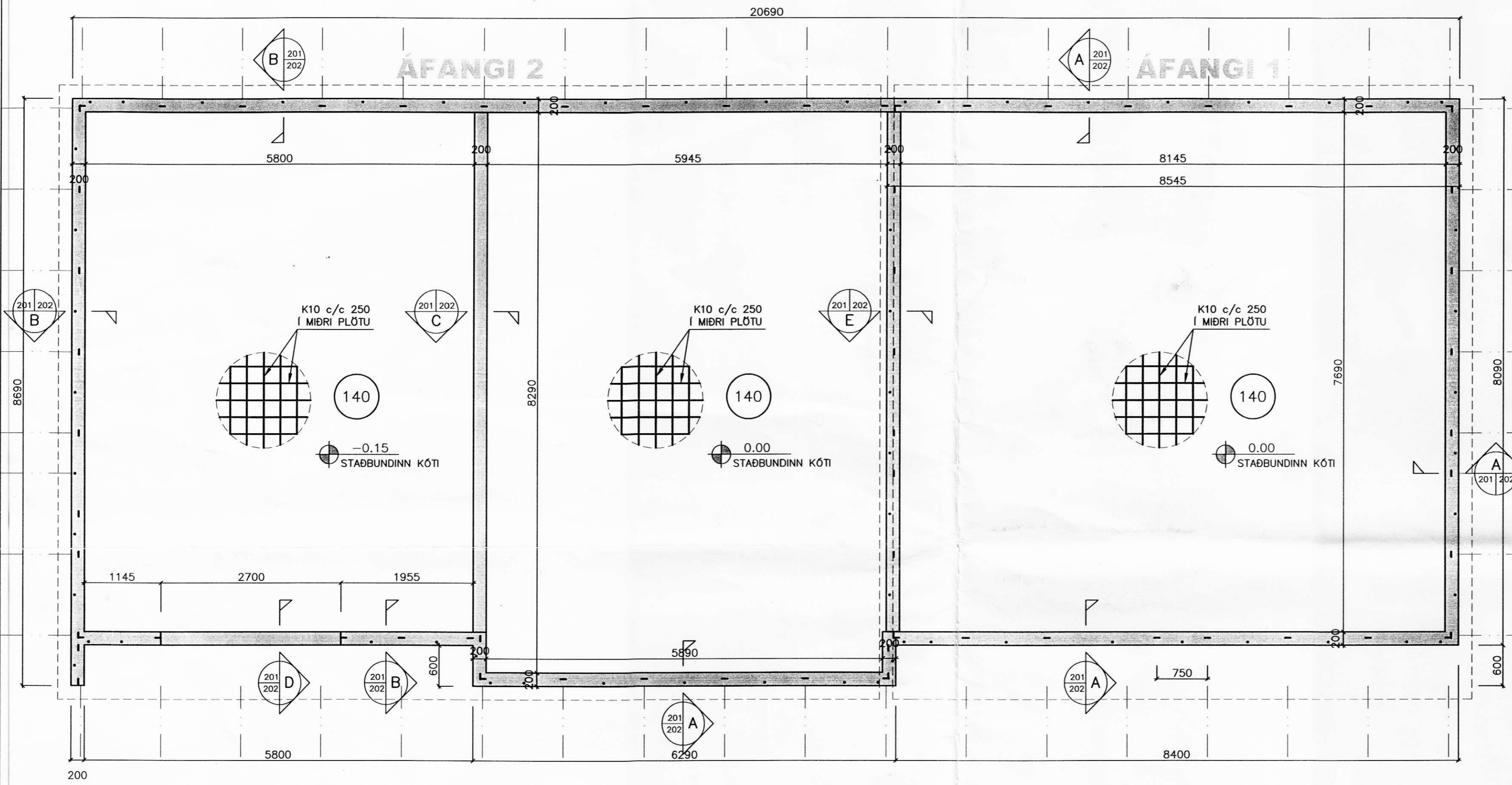
GRUNNMYND SÖKKULS Mkv. 1:50
