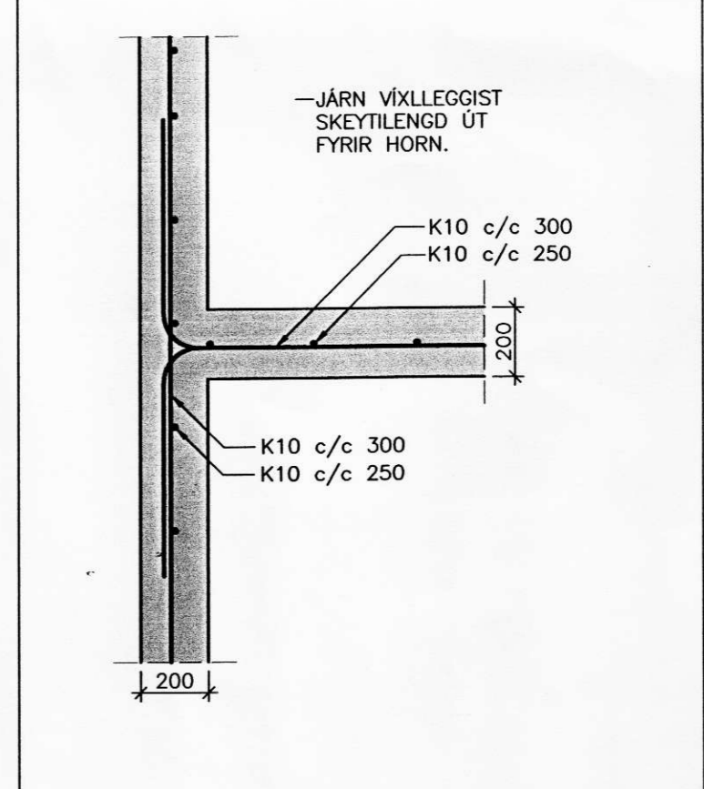
LÄRÉTT SNID Í SÖKKULVEGG Mkv. 1:20
