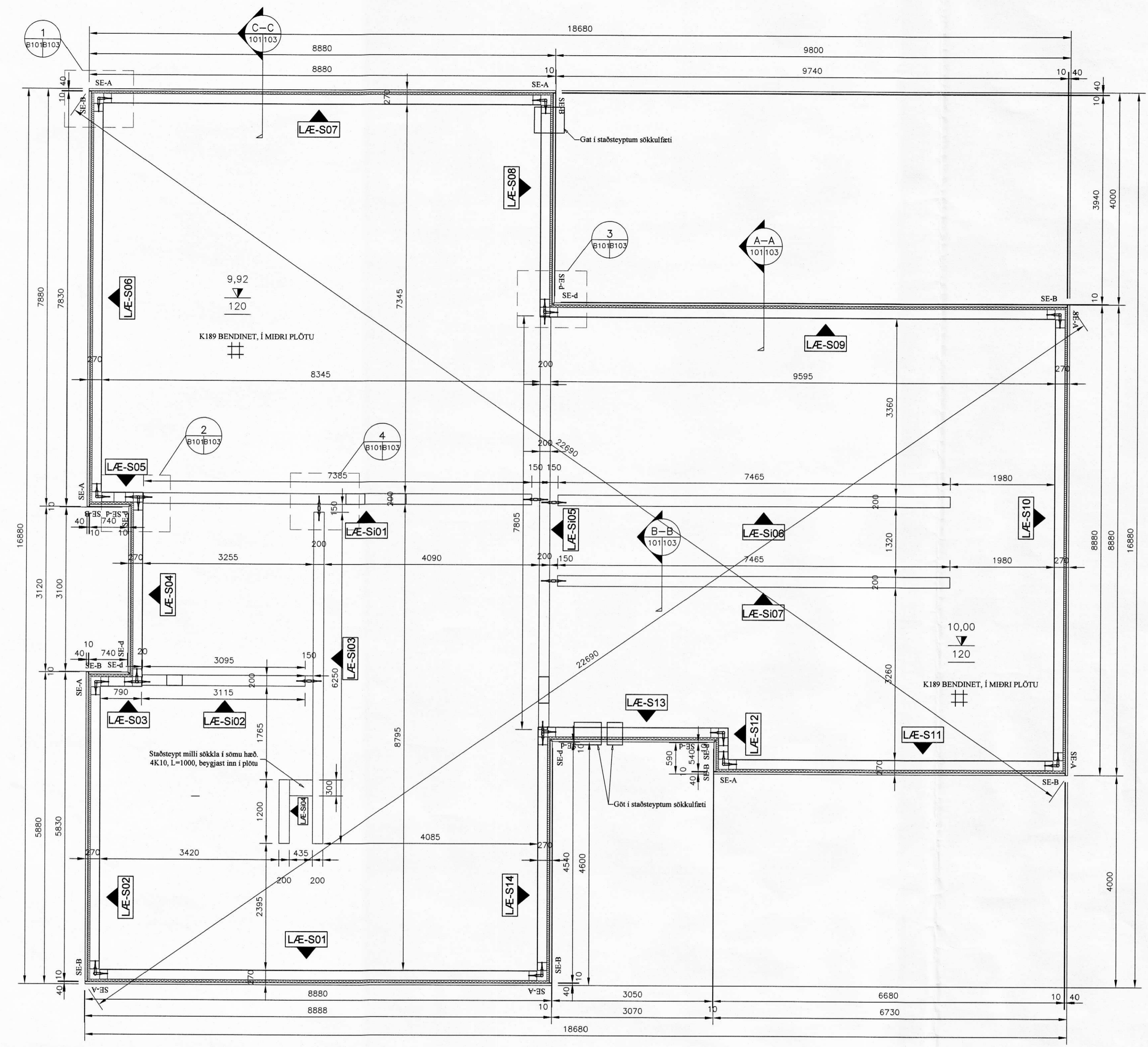
GRUNNMYND - SÖKKLAR 1:50
