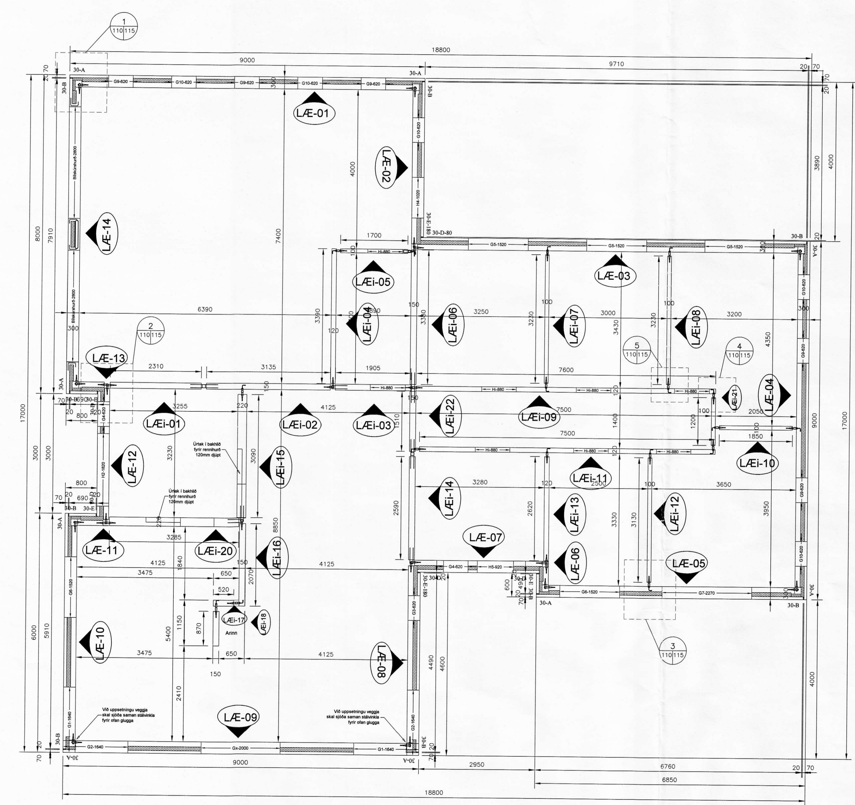
GRUNNMYND 1:50
