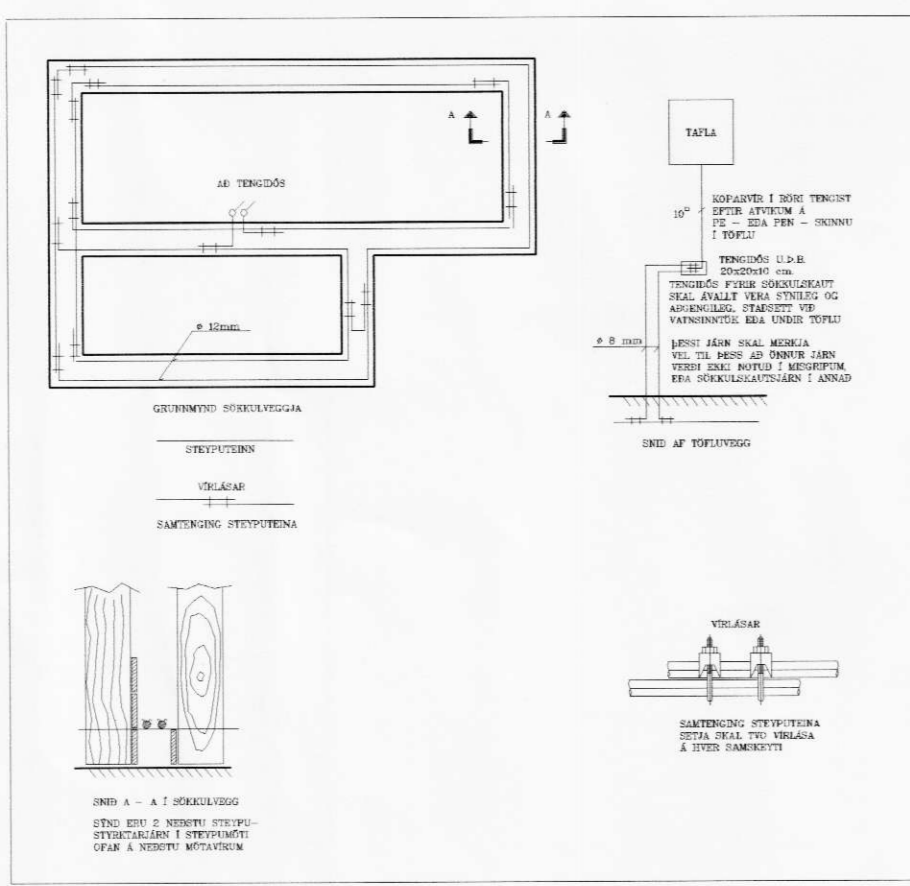
SKYRINGAMYNDIR AF SOKKULSKAUTI ERU EKKI Í MELIKVARÐA
