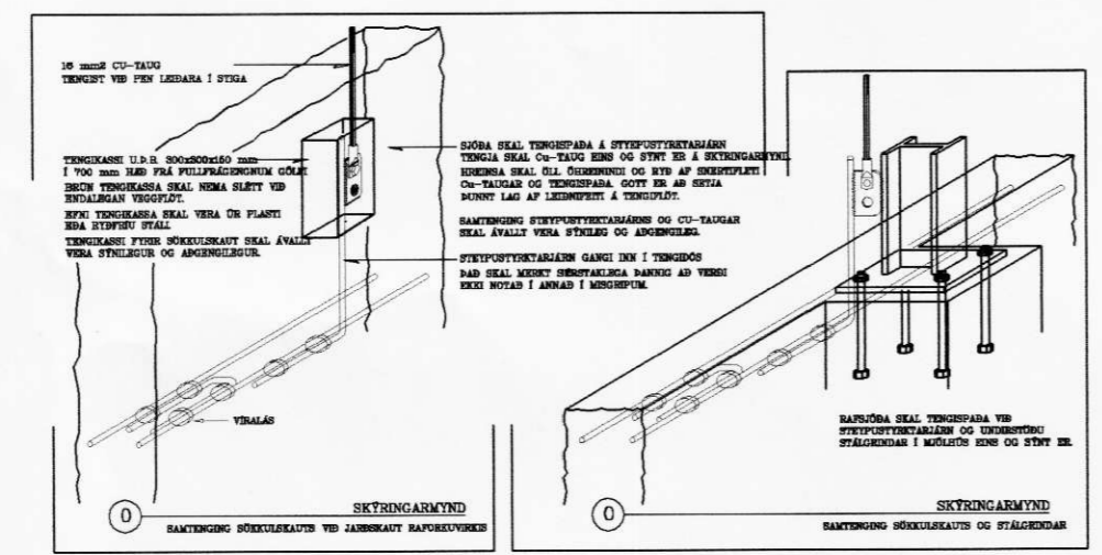
ATHUGIÐ: SKYRINGAMYNDIR AF SOKKULSKAUTI ERU EKKI Í MELIKVARÐA
