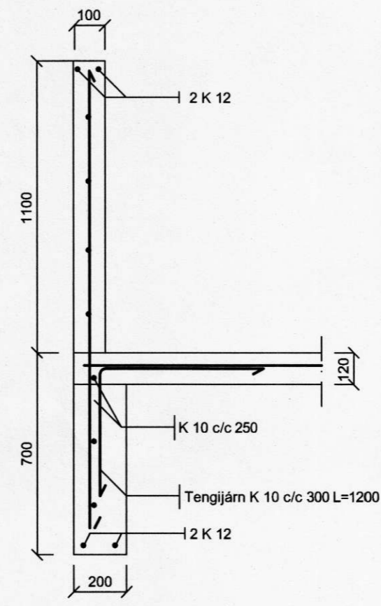
Mkv. 1:20 K B-01a-b
