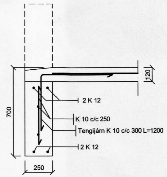
Mkv. 1:20 G B-01a-b
