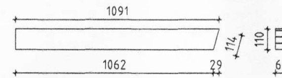
T1 - 65x110 Mkv 1:20 Samtals 4 stk
