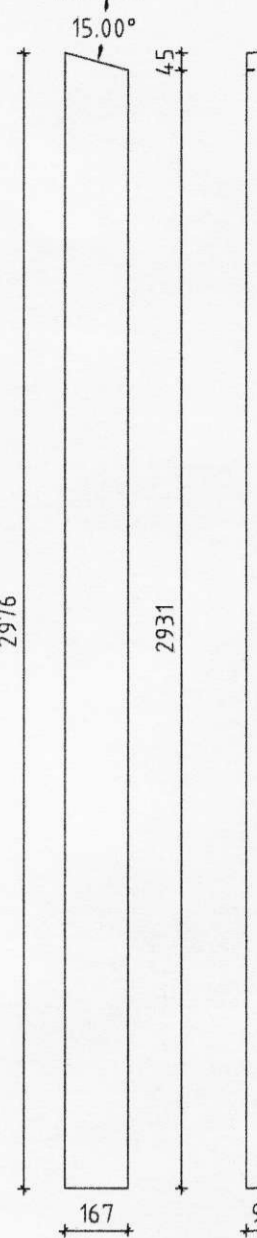
VS3 - 90x167 Mkv 1:20 Samtals 4 stk
