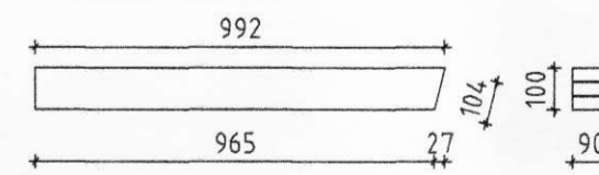
T3 - 90x100 Mkv 1:20 Samtals 4 stk
