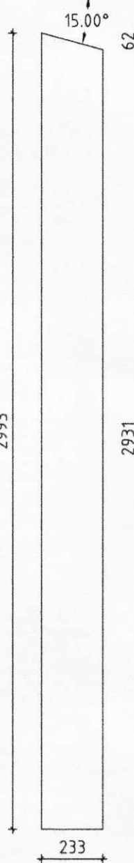
VS2 - 115x233 Mkv 1:20 Samtals 8 stk
